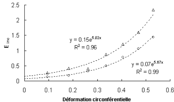
FIG. 4.10 – Modules d'élasticité incrémentaux. Les ronds correspondent aux échantillons frais et les triangles aux échantillons cryoconservés.
