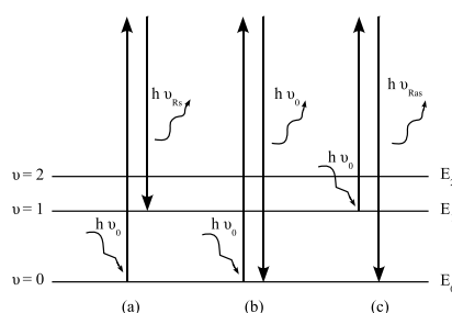
FIG. 1.10 – (a) Diffusion Raman Stokes ( \nu_{R_s} = \nu_0 - \nu_a ), (b) Diffusion élastique, (c) Diffusion Raman anti-Stokes ( \nu_{R_{as}} = \nu_0 + \nu_a ), avec \nu_0 la fréquence de la source monochromatique excitatrice du spectre. Si le photon incident a une énergie très supérieure au niveau d'énergie de vibration, alors on observe un phénomène de diffusion :
