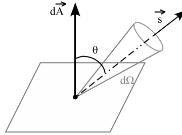
FIG. 3.12 – Espace des grandeurs utilisées.
