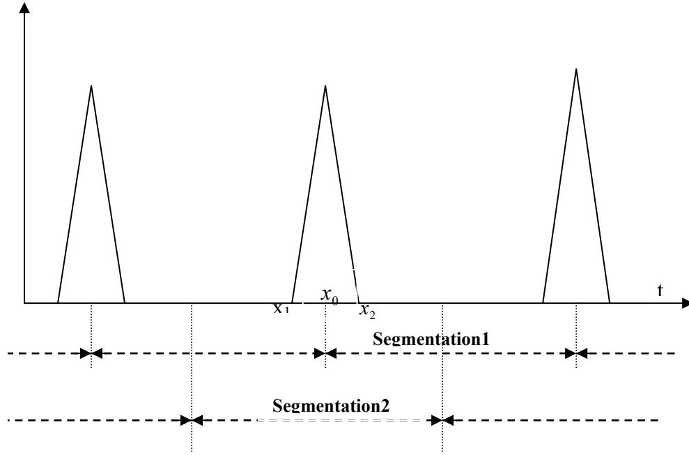
Figure 3-6 : Modèle simplifié du signal ECG servant à déterminer théoriquement le choix de la segmentation. [Philips 92] ( \delta_1 = x_0 - x_1 et \delta_2 = x_2 - x_0 ).
