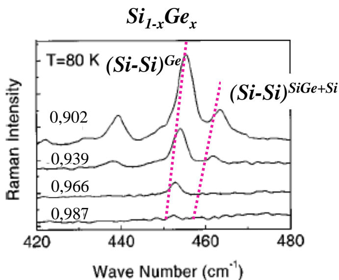
Figure-4-12 (Franz, et al., 1999) Spectres Raman enregistrés sur des cristaux massifs de Si_{1-x}Ge_x à basse température (80K) dans la gamme spectrale (Si-Si). Le labelling des modes est celui proposé par nos soins dans le cadre du modèle de percolation. Cette situation correspond à l'ovale 1 dans la Figure-4-11 .
