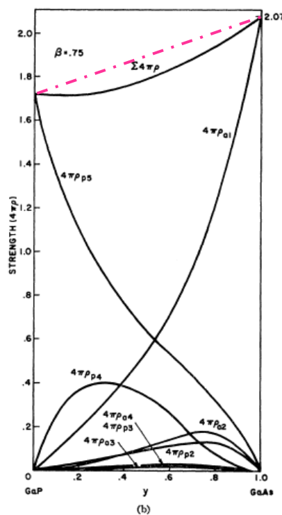
Figure-3-13 Forces d'oscillateurs en fonction de la composition ( y ) calculée à partir du modèle de VB pour \beta = 0,75 . On remarque que la force d'oscillateur par alliage, déduite en sommant sur les liaisons Ga-As et Ga-P ne varie pas linéairement avec la composition de l'alliage. En fait elle est sous-estimée de façon significative. Figure prise de la référence (Verleur et Barker, 1966). La droite en pointillée est ajoutée pour la comparaison.
