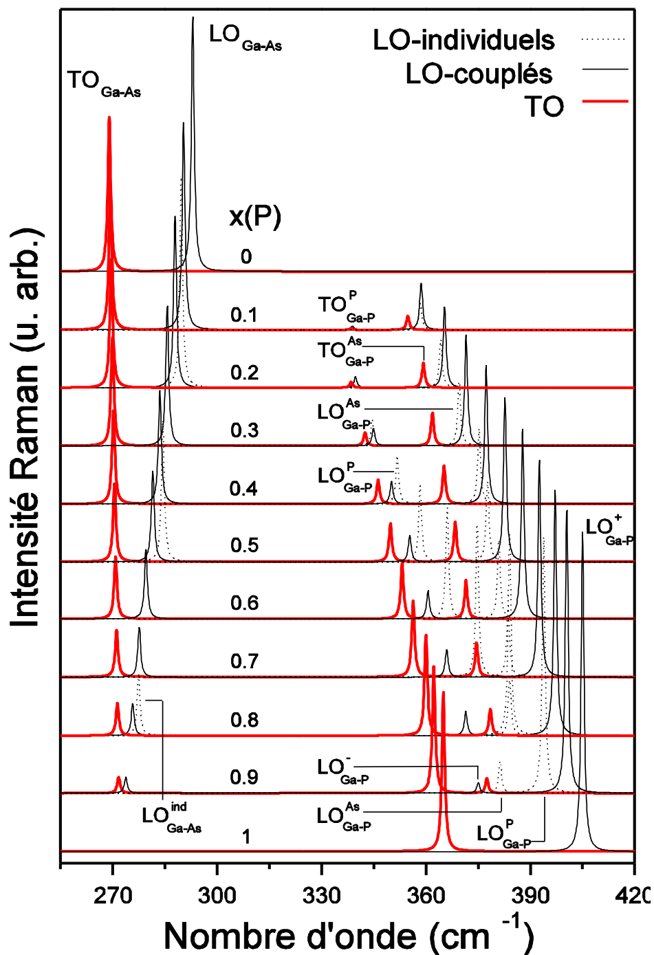
Figure-3-5 Courbes Raman TO (traits rouges épais), LO-couplés (traits fins) et LO-individuels (pointillés) calculées pour l'alliage \text{GaAs}_{1-x}\text{P}_x aléatoire à l'aide de l'équation (2.32) du chapitre 2 en utilisant les fréquences TO et fractions d'oscillateurs indiquées en Figure-3-3 . Un amortissement phonon \gamma faible, de 1\text{cm}^{-1} , est utilisé pour tous les oscillateurs et à toutes les compositions x .
