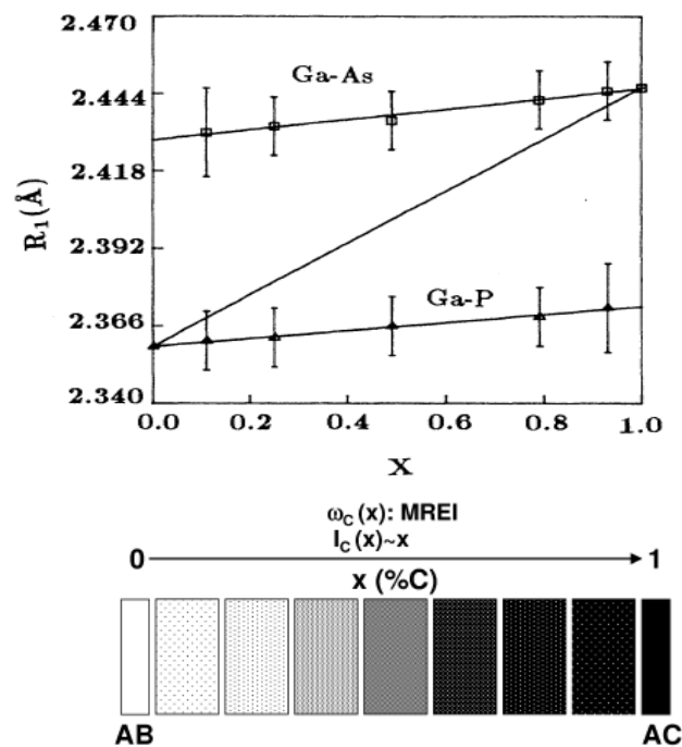
Figure-0-2 Haut : (Wu, et al., 1993) Données EXAFS relatives aux distances premiers-voisins (longueurs de liaisons) dans GaAsP . Bas : Tout se passe comme si, à une composition donnée, les liaisons chimiques d'un type donné sont toutes plongées dans le même continuum uniforme à propriétés physiques lentement variables en fonction de la composition selon l'approximation du cristal virtuel (voir le dégradé de gris du milieu hôte des liaisons chimiques).
