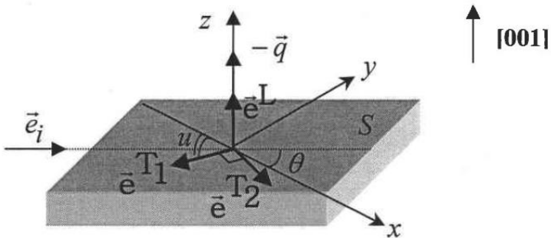
Figure-2-4 Dans le cas de la rétrodiffusion, configuration des vecteurs \vec{e}^{T_1} , \vec{e}^{T_2} , \vec{e}^L , \vec{e}_i par rapport au vecteur d'onde q des phonons parallèle à l'axe x[100] du cristal cubique.
