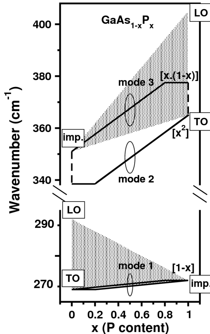
Figure-3-14 Vue schématique du comportement 1-liaison → 2-TO de percolation (traits épais) pour GaAsP . Les fractions d'oscillateurs individuels TO sont indiquées entre crochets. Les segments obliques de type MREI-renormalisé sont simplifiés par des droites, pour plus de clarté. L'analogie avec les schémas de percolation des systèmes de type InGaAs , ZnTeSe et InGaP représentant les trois variantes admises du type MREI (cf. figure Figure-2-18 du chapitre 2), est claire.
