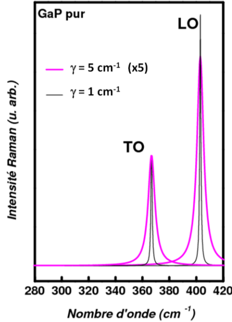
Figure-2-3 Courbes Raman TO et LO du GaP pur calculées en utilisant l'équation (2.31) pour des amortissements phonons de \gamma = 1 \text{ cm}^{-1} et \gamma = 5 \text{ cm}^{-1} .
