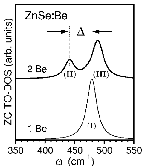
Figure-2-16 Densités d'états des phonons projetés à q=0 relatifs au Be pour 1 (bas) et 2 (haut) atomes de Be posés dans une supercellule de type ZnBe (64 atomes).
