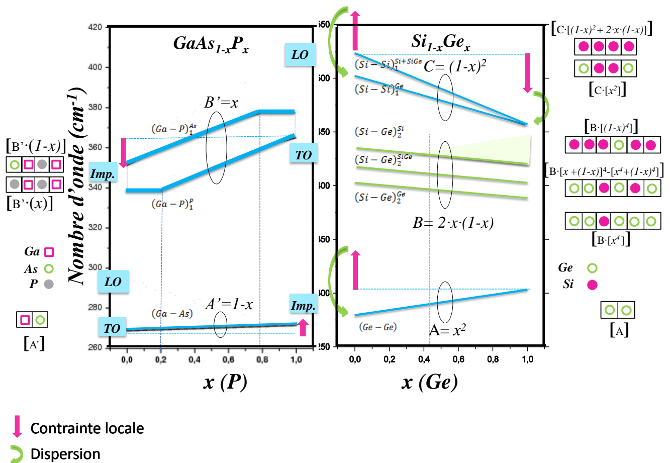
Figure-5- 2 Comparaison schématique des schémas de percolation TO de GaAsP (zincblende, basé sur l'effet de contrainte locale seulement) et de SiGe (diamant, avec effets conjoints de la contrainte locale et de la dispersion phonon).
