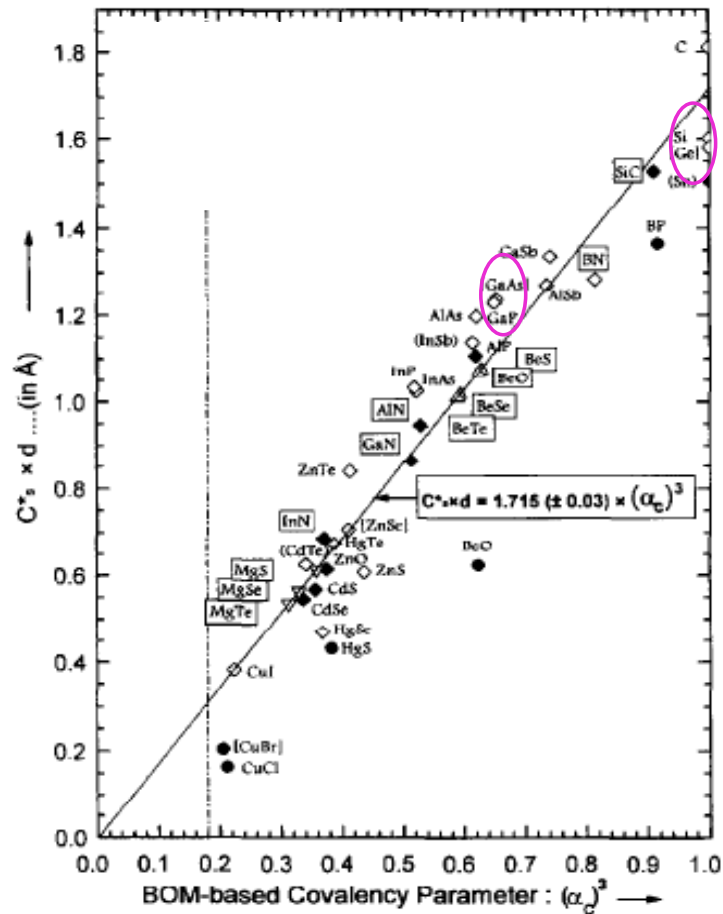
Figure-0-1 (Vèrié, 1998). Produit C_s^*d entre le module de cisaillement réduit ( C_s^* ) et la longueur de liaison ( d ) en fonction de la covalence ( \alpha_c^3 ) de la liaison chimique. Plus on s'éloigne de la colonne IV du tableau périodique, plus C_s^*d est faible. SiGe et GaAsP semblent constituer des alliages idéaux puisque le contraste entre les valeurs C_s^*d des parents est quasi nul (cf. ovales).
