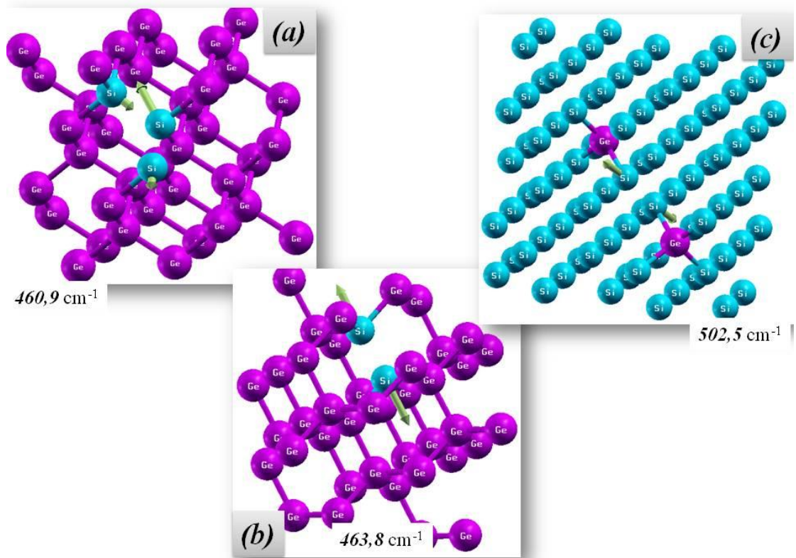
Figure-4-7 (a) Supercellule de type 'Ge' contenant trois impuretés Si quasi-alignées, donnant accès au stretching Si-Si en environnement (1) mixte (Si, Ge) de type ACL. (b) supercellule de type 'Ge' contenant une liaison Si-Si unique, donnant accès au stretching de la liaison isolée Si-Si, en présence de Ge. (c) supercellule de type 'Si' contenant deux impuretés Ge en positions troisièmes voisins, donnant accès au mode de stretching Si-Si en environnement tout-Ge dans la limite diluée en Ge.
