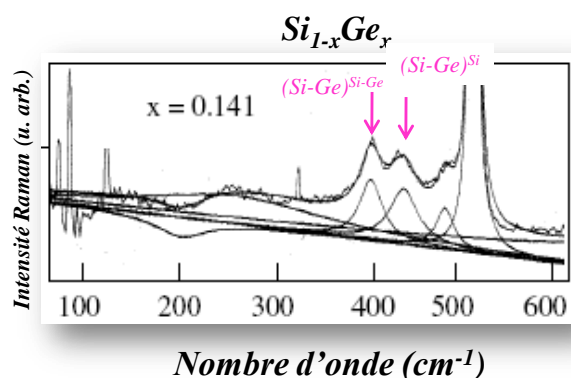
Figure-4-15 Spectres Raman enregistrés avec Si_{1-x}Ge_x par (Rath, et al., 2003) dans la limite d'une incorporation faible de Ge dans la gamme spectrale Si-Ge. On note la quasi-égalité des intensités entre le mode central (Si-Ge)^{SiGe} (qui domine à composition intermédiaire) et son pic satellite (Si-Ge)^{Si} (à plus haute fréquence). Cette situation correspond à l'ovale 3 dans la Figure-4-11.
