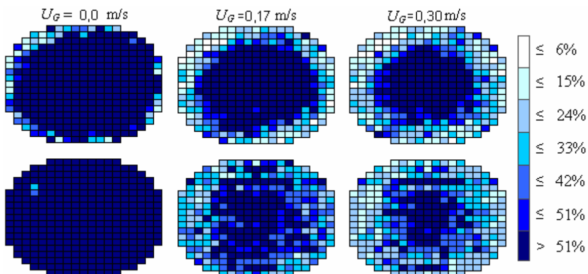
Figure 3-37 Distributeur central : Images obtenus pour un lit de particules en PE à U_L = 0,0082 \text{ m/s} pour différents débits de gaz.
