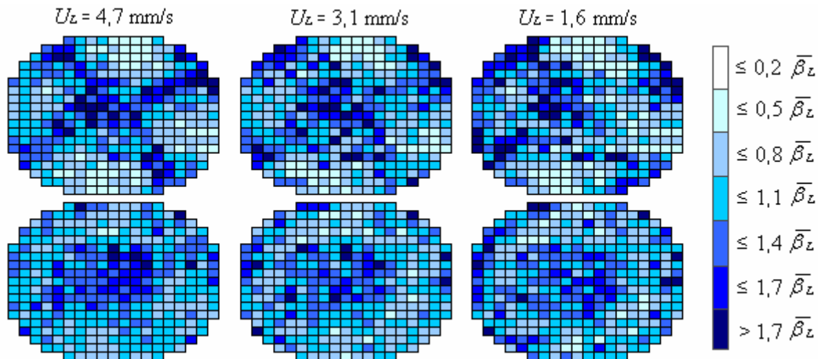
Figure 3-16 Résultats obtenus pour un chargement sock à U_G \approx 0,17 m/s et à différents débits de liquide.
