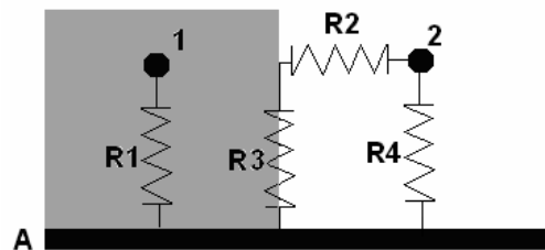
Figure 2-25 Représentation de la Figure 2-24 sous la forme d'un circuit électrique.
