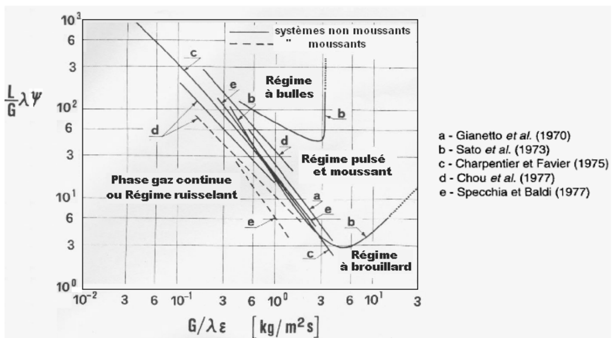
Figure 1-2. Gianetto et coll. (1978): Cartes d'écoulement proposées par différents auteurs selon les coordonnées de Gianetto et coll. (1978)
