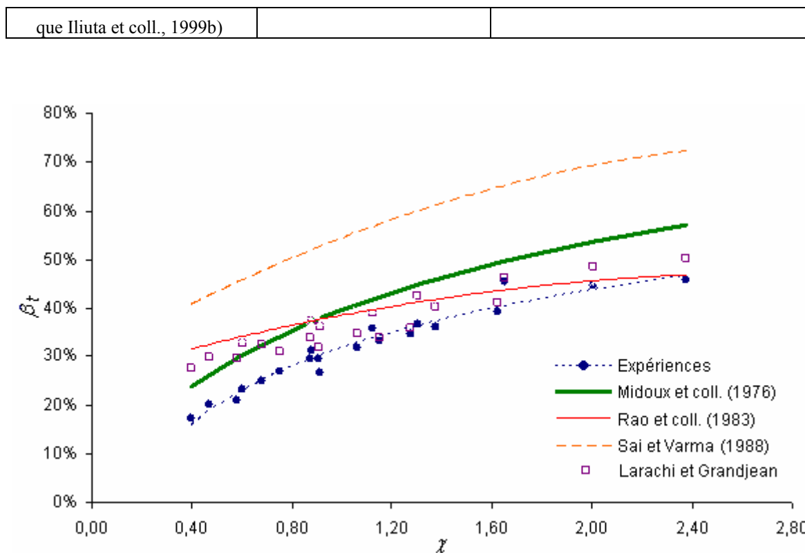
Figure 3-32 Evolution de la saturation de liquide totale pour un lit d'extrudés en PE en fonction de \chi .
