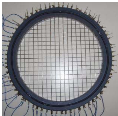
Figure 2-27 Système de tomographie à fils.
