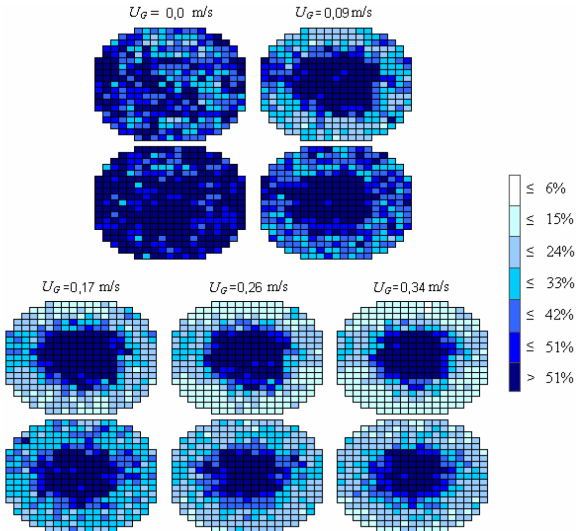
Figure 3-20 Distributeur central : Images obtenues pour un chargement sock à U_L = 0,0082 m/s pour différents débits de gaz.
