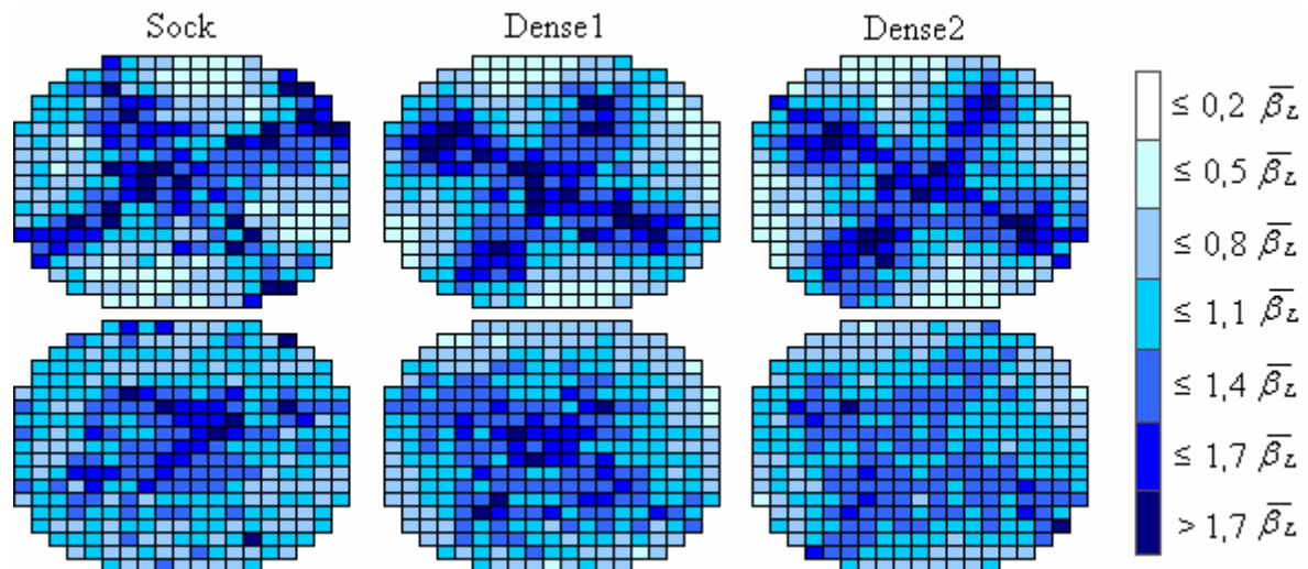
Figure 3-19 Images obtenues par tomographie à fils pour les trois chargements étudiés à U_L = 0,0064 m/s et U_G = 0,17 m/s.
