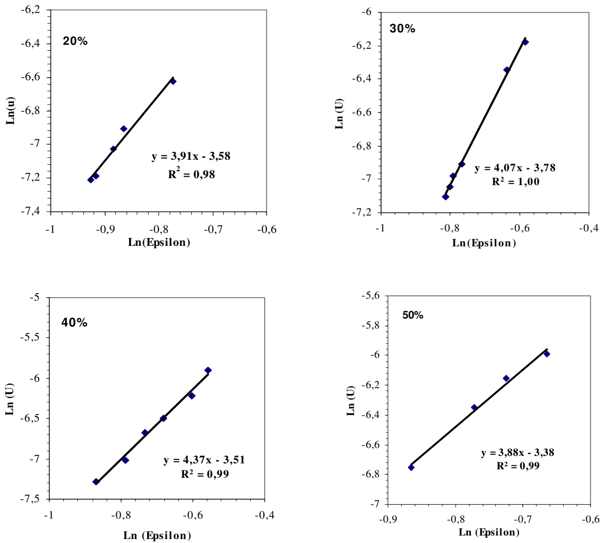
Fig. (IV-7) : \ln(U) = f(\ln(\epsilon)) pour des billes de diamètre 105-200 \mu\text{m} à différents pourcentages massiques
