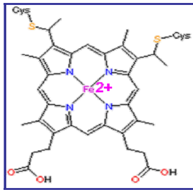
Figure 14 : Représentation schématique d'un hème de type c et de sa fixation au sein d'un cytochrome c. L'hème est relié aux deux Cys de l'apocytochrome c via deux liaisons thioéthers impliquant les groupements vinyloxy de l'hème. L'atome de Fe^{2+} est coordonné par quatre noyaux pyroles et par His de l'apocytochrome c et appartenant à la signature CXXCH (non figuré sur le schéma).
