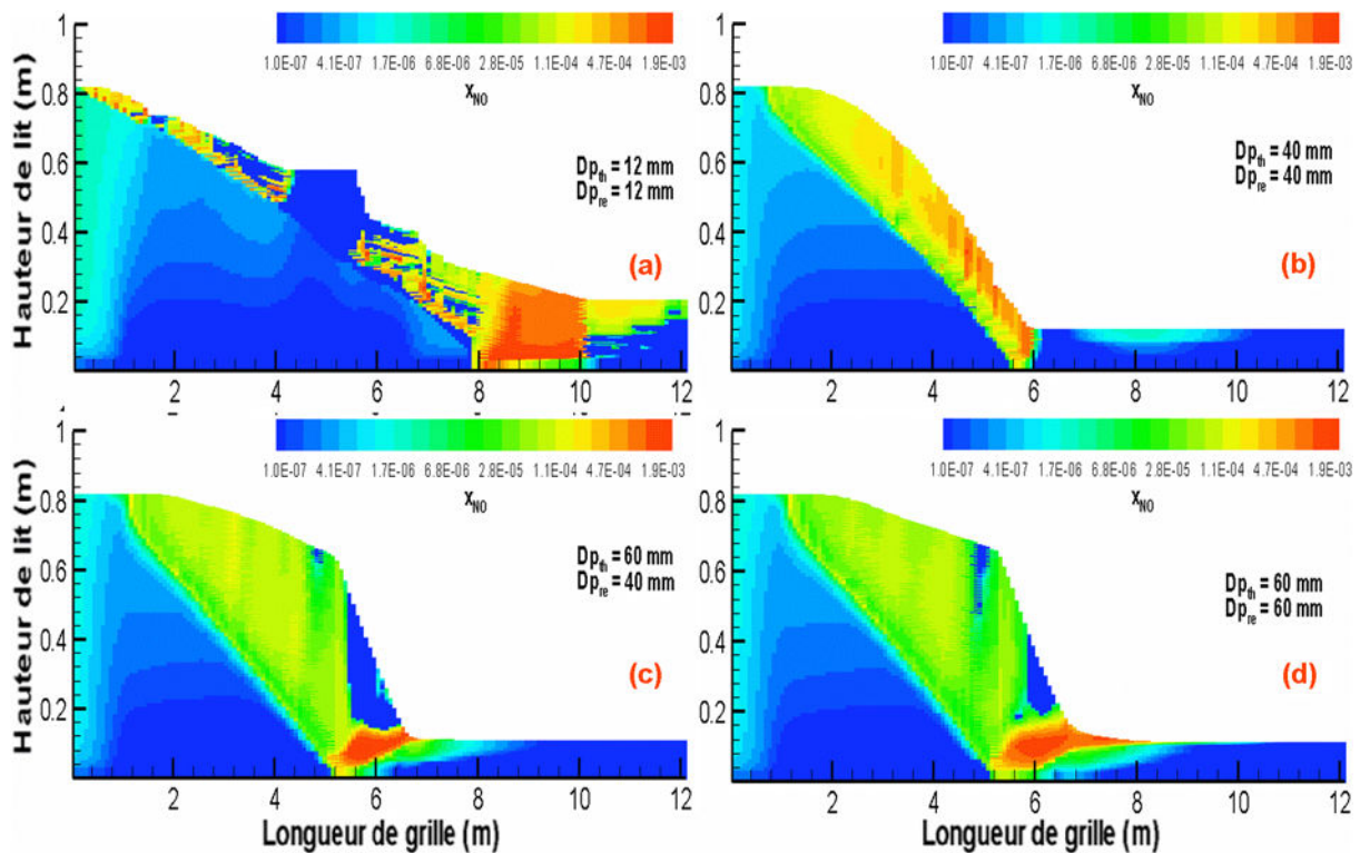
Figure 4.20. Influence du diamètre des particules d'OM sur le titre molaire en \text{NO}
