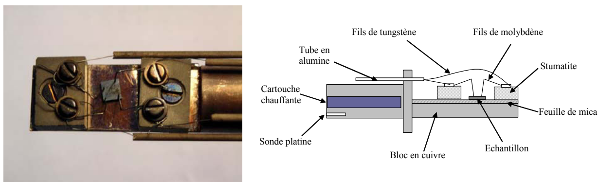
(a) (b) Figure 51 : Photographie (a) et schéma (b) de la cellule de mesure de la résistivité électrique à haute température
