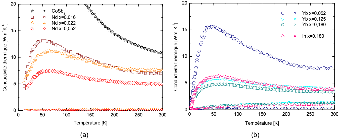
Figure 70 : Dépendance en température de la conductivité thermique de réseau et de la conductivité thermique électronique pour les composés R x Co 4 Sb 12 : R = Nd (a) et R = Yb, In (b)
