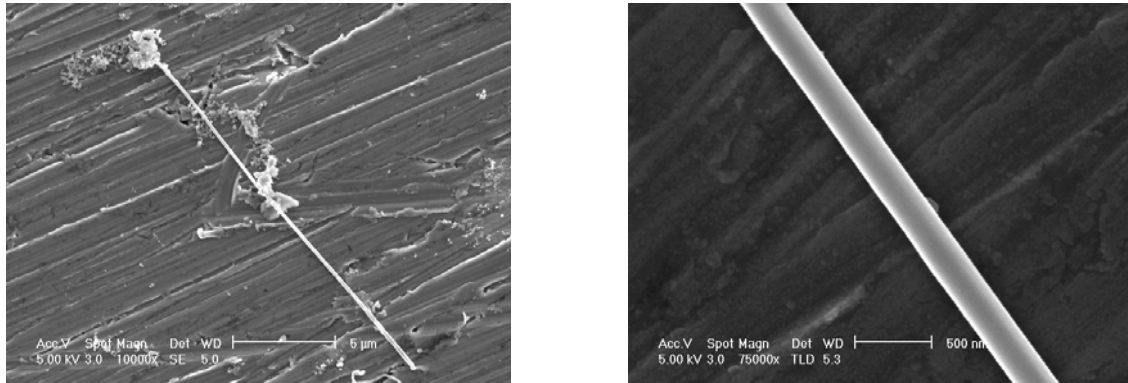
Figure III.21 Images MEB de nanotubes ou de nanobarreaux obtenus lors de l'interaction du faisceau laser avec les poudres micrométriques dans la cellule dédiée à la synthèse de nanopoudres ( \lambda = 532 \text{ nm} , D = 27 \text{ cm} , 1 h, matériau de type p, 300 mJ en sortie).
