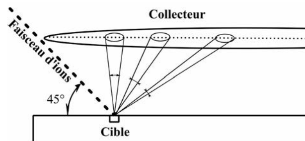
FIG. I.6 - Variation de l'angle solide en fonction de la position du diaphragme.
