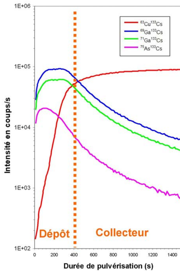
FIG. III.7 - Profil en profondeur d'un dépôt de GaAs sur le collecteur de Cu. La ligne orange désigne l'estimation de l'interface entre le dépôt et le collecteur.
