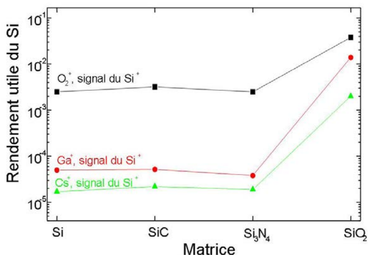
FIG. I.2 - Rendement utile (le nombre de particules détectées par atome émis hors de la cible) du Si en fonction de la cible et de l'ion primaire [2]. Nous constatons que le rendement utile du Si + dans le SiO 2 est très largement supérieur. Celui-ci varie proportionnellement à la probabilité d'ionisation. L'augmentation de signal est une conséquence de l'effet de matrice.
