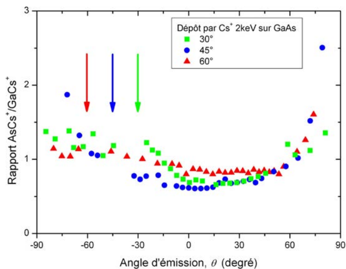
FIG. IV.30 - Evolution du rapport des signaux \text{AsCs}^+ et \text{GaCs}^+ en fonction de l'angle d'émission pour trois angles d'incident du faisceau. Les flèches indiquent la direction du faisceau d'ions pour chaque angle d'incidence. Le rapport est normalisé tel que sa valeur moyenne soit égale à 1.
