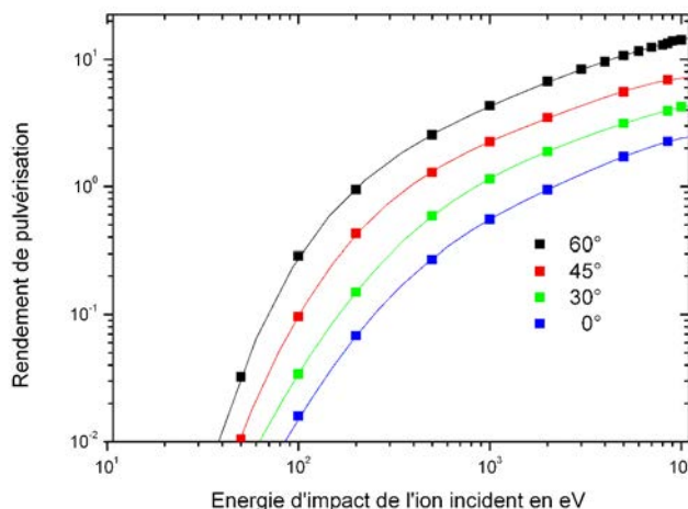
FIG. IV.2 - Calculs numériques du rendement de pulvérisation du Si par des ions Cs + en fonction de l'énergie d'impact.
