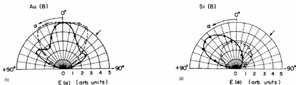
FIG. II.22 - Distribution angulaire de l'Au (220) (à gauche) et du Si (100) (à droite) pour un bombardement d' Ar^+ avec une incidence de 45^\circ et une énergie d'impact de 1 keV. Dans le cas de l'or, la distribution angulaire dépend des directions préférentielles du cristal tandis que le silicium ne semble pas en dépendre [74].
