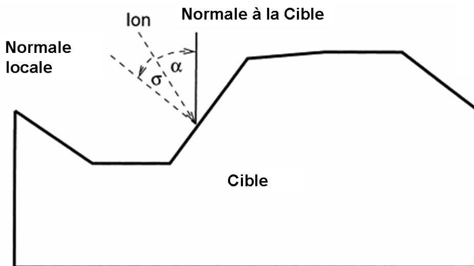
FIG. II.12 - Schéma de l'effet de la rugosité sur l'angle d'incidence locale. L'angle \sigma entre le faisceau incident et la normale locale diffère de l'angle fait par rapport la normale à la surface de la cible \alpha . [31]
