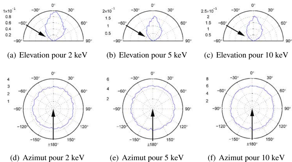
FIG. IV.5 - Les distributions angulaires dY/d\Omega du Si par des ions Cs^+ en fonction de l'énergie avec un angle d'incidence de 60^\circ en atomes/ion.sr. La flèche noire représente le faisceau incident. Nous pouvons observer que les distributions en élévation a) b) et c) sont de type sur-cosinus. Les distributions en fonction de l'azimut sont quasi circulaires. Pour 2 keV a) et d), nous pouvons observer un léger déplacement de la distribution dans la direction spéculaire au faisceau incident.
