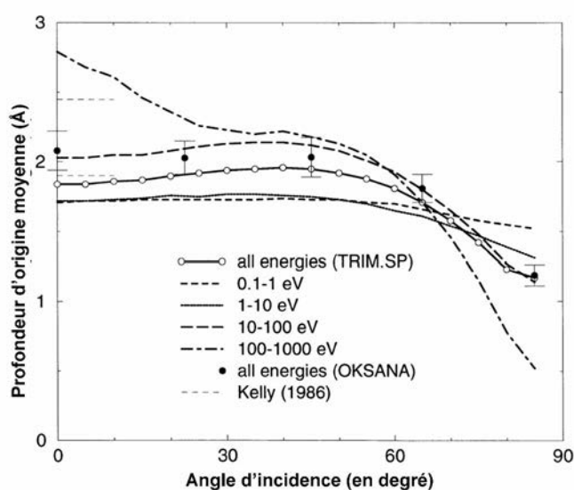
FIG. II.17 - Profondeur d'origine moyenne en fonction de l'angle d'incidence pour une cible de Si bombardée par des ions \text{Ar}^+ avec une énergie d'impact de 1 keV [61].
