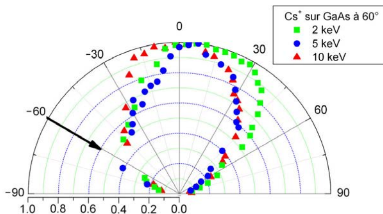
FIG. IV.27 - Distribution angulaire globale du GaAs pour un bombardement d'ions primaires de \text{Cs}^+ avec un angle d'incidence de 60^\circ par rapport à la normale à la surface en fonction de l'énergie d'impact. La flèche noire indique la direction du faisceau d'ions incident.
