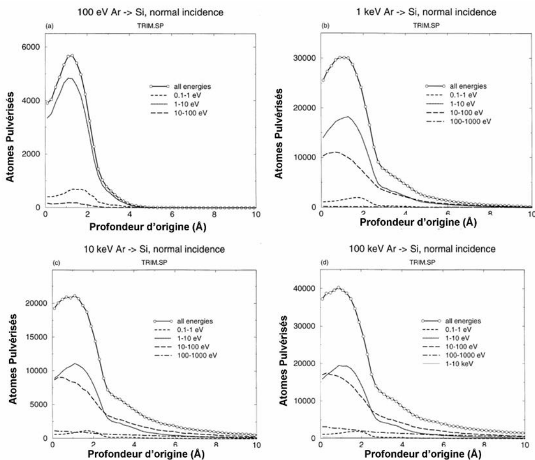
FIG. II.16 - Distribution des atomes de Si pulvérisés par des ions Ar^+ en fonction de leur profondeur d'origine et de la gamme d'énergie de l'atome émis pour quatre énergies d'impact différentes et à incidence normale par rapport à la surface [61].
