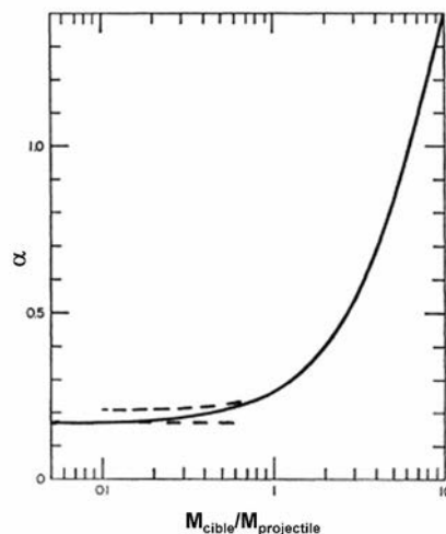
FIG. II.7 - Evolution du paramètre \alpha en fonction du rapport des masses de l'atome cible et du projectile.[18]
