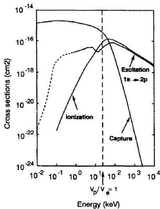
FIG. II.4 - Section efficace des processus inélastiques en fonction de la vitesse du projectile par rapport à la vitesse de Bohr. Cas d'un proton sur un atome d'H [15].
