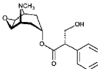
Scopolamine Formule : C_{17}H_{21}NO_4 Masse de Mol : 303,4g
