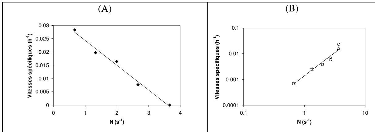
Figure IV-17 : Corrélations de la vitesse d'agitation (N, en \text{s}^{-1} ) avec les vitesses spécifiques de croissance et de mort cellulaire de CHO cultivées sans pluronic et en spinner : (A) \mu_{app} (◆), et (B) k_l (○) et k_d (△).
