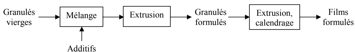
Figure 2.1. Schéma du processus de mise en forme des films formulés étudiés.
