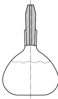
Figure 2.2. Pycnomètre de Gay-Lussac
