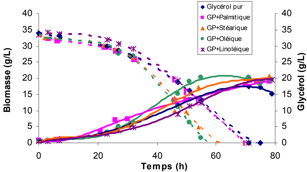
Figure III.18. Cinétiques de croissance et de consommation du glycérol pur de SP. ruberrimus à 23 °C, pH 6 et OD = 50 %. Cultures réalisées avec ajout de différents acides gras (palmitique, stéarique, oléique et linoléique) à une même concentration de 2 g/L.
