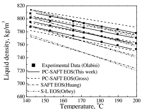
图3.12 聚乙烯液相密度比较
