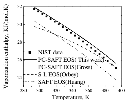
图3.9 己烷摩尔蒸发焓的比较
