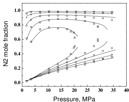
图3.17 氮气-己烷体系的汽液平衡计算值和文献值 [696] 比较
