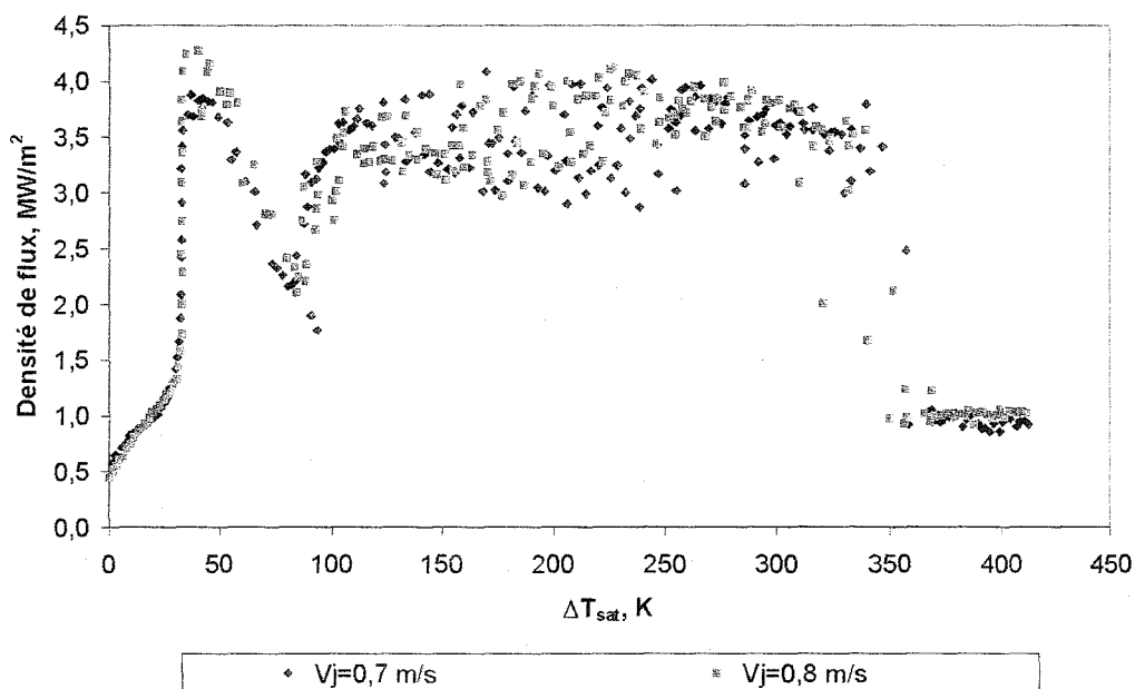
FIG. 3.25 – Influence de la vitesse à l'impact, Robidou [2000]
