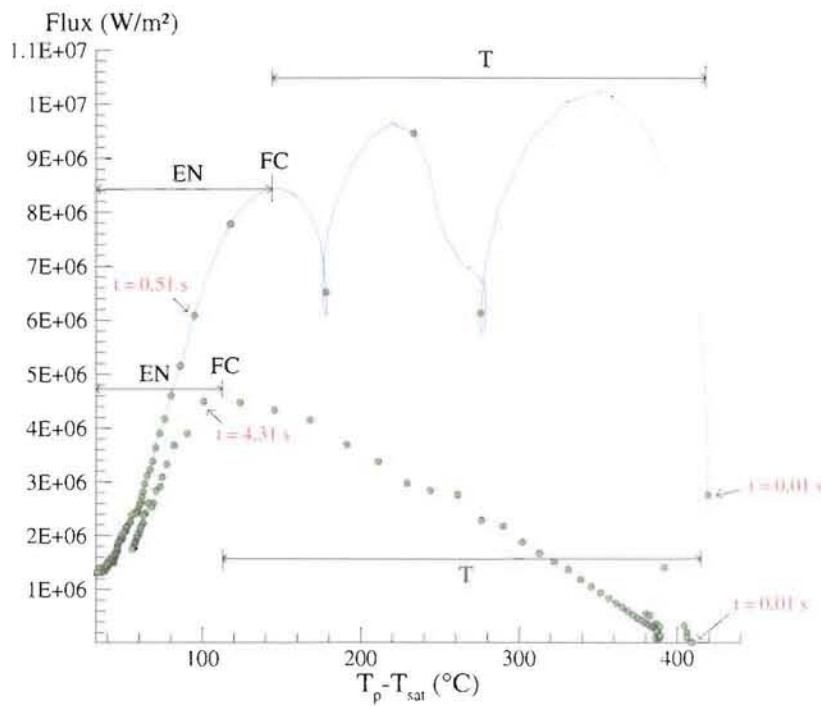
FIG. 4.17 – Courbes d'ébullition locales, à l'impact (courbe bleue) et à 1,5 cm de l'impact (courbe rose); \Delta T_{sub} = 80K et V_j = 1,20 m/s; EN : Ebullition Nucléée, FC : Flux Critique, T : régime de Transition
