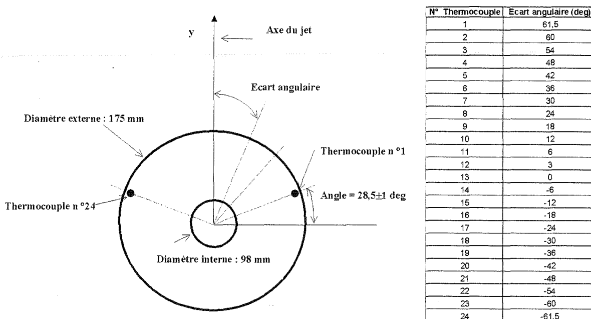
FIG. 4.2 – Répartition angulaire des thermocouples.
