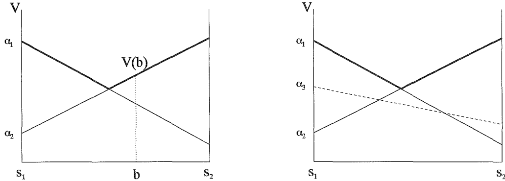
FIG. 1.2 – La fonction de valeur d'un POMDP à deux états s_1 et s_2 . L'action associée au vecteur \alpha_2 correspond à l'action optimale en b . Le vecteur \alpha_3 est entièrement dominé et peut être supprimé sans affecter la représentation de la fonction de valeur optimale.
