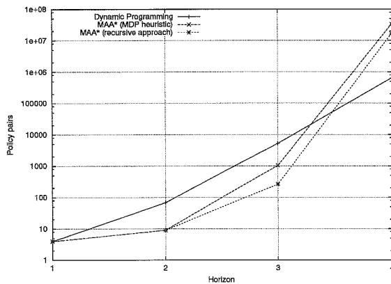
FIG. 1.7 – Le nombre de politiques évaluées pour l'approche de programmation dynamique, MAA* avec l'heuristique MDP et MAA* avec l'heuristique récursive pour le problème du réseau de communication (échelle logarithmique).
