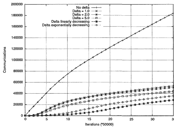
FIG. 1.12 – Le nombre total de communications effectuées pour 3 seuils fixes différents, deux seuils variables et le cas sans seuil.
