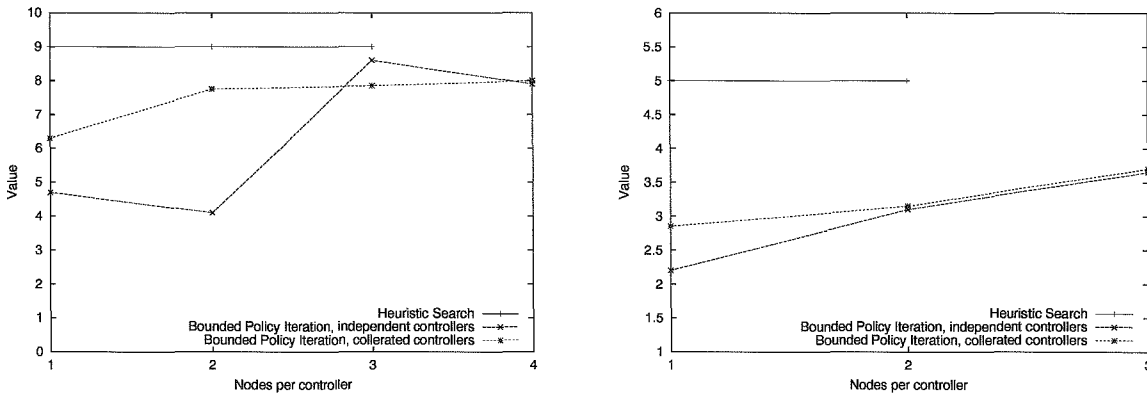
FIG. 1.9 – Valeur optimale des politiques déterministes pour l'approche de recherche heuristique, comparée à deux évaluations de bounded policy iteration pour des contrôleurs stochastiques tirées de [BHZ05]. A gauche : Réseau de communication - A droite : Rencontre sur une grille.
