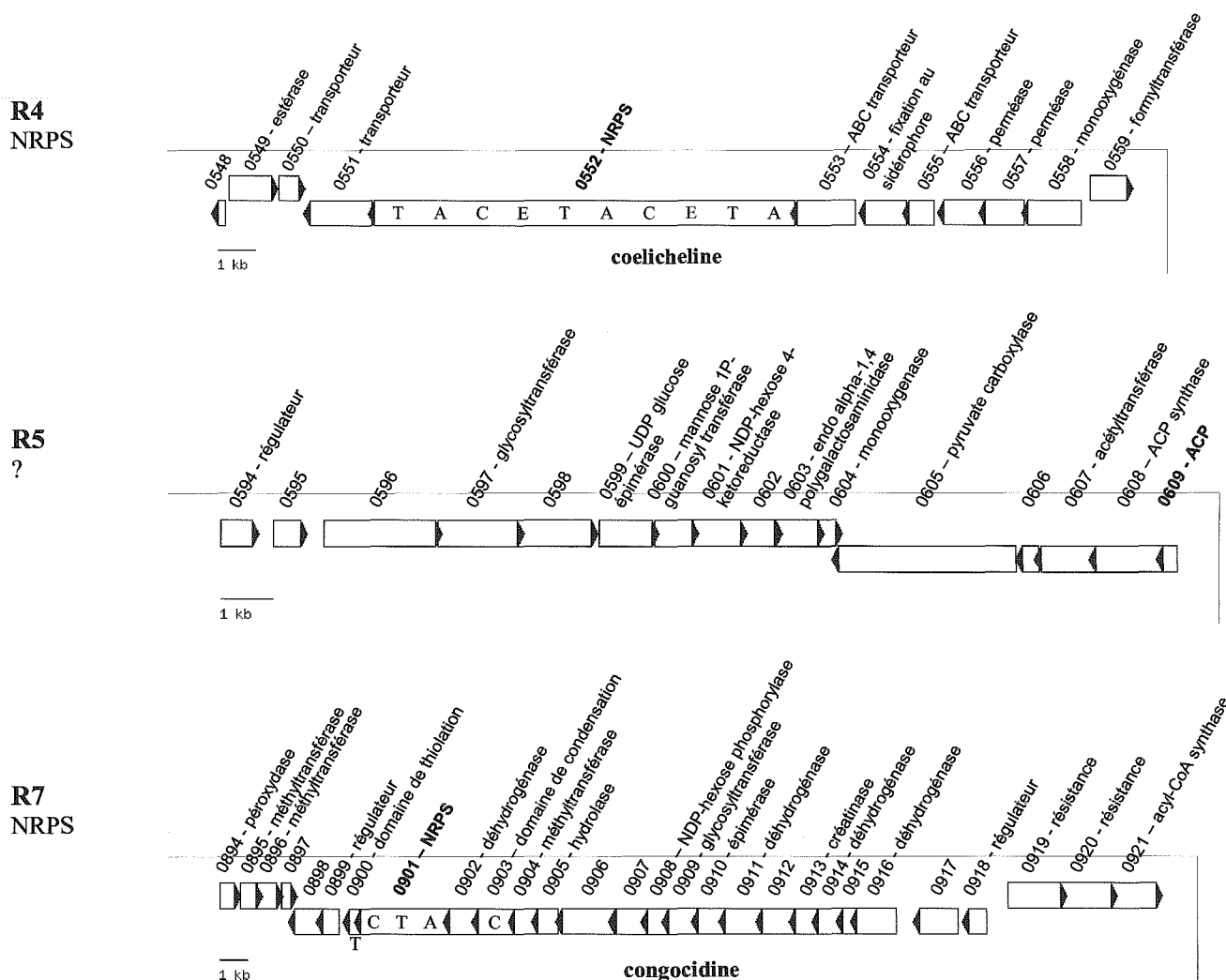
Figure 32 : Schéma des clusters potentiellement impliqués dans la biosynthèse de métabolites secondaires chez S. ambofaciens . Les numéros correspondent aux noms des gènes sans le préfixe "SAM[LR]".
