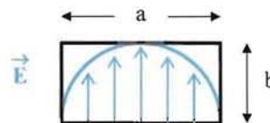
Figure 66 : Orientation du champ électrique dans la section du guide
