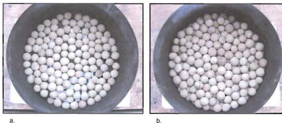
Figure 120 : Lit filtrant de 1 cm (a) et 2 cm (b)
