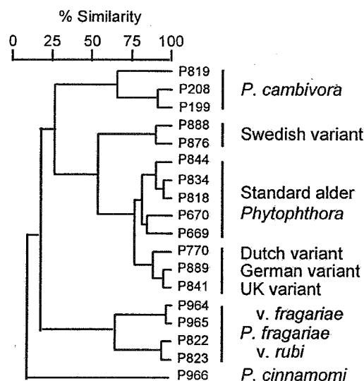
Figure 4 : Dendrogramme construit à l'aide de l'algorithme UPGMA (Unweighth Pair Group Method with Arithmetic mean) à partir d'empreintes AFLP générées à partir de l'ADN total d'isolats de Paa (ex « standard type»), Pam (ex « Dutch, German, and UK variant »), Pau (ex « Swedish variant »), P. cambivora et P. fragariae sensu lato . P. cinnamomi a été utilisé comme groupe externe. Extrait de Brasier et al. (1999).
