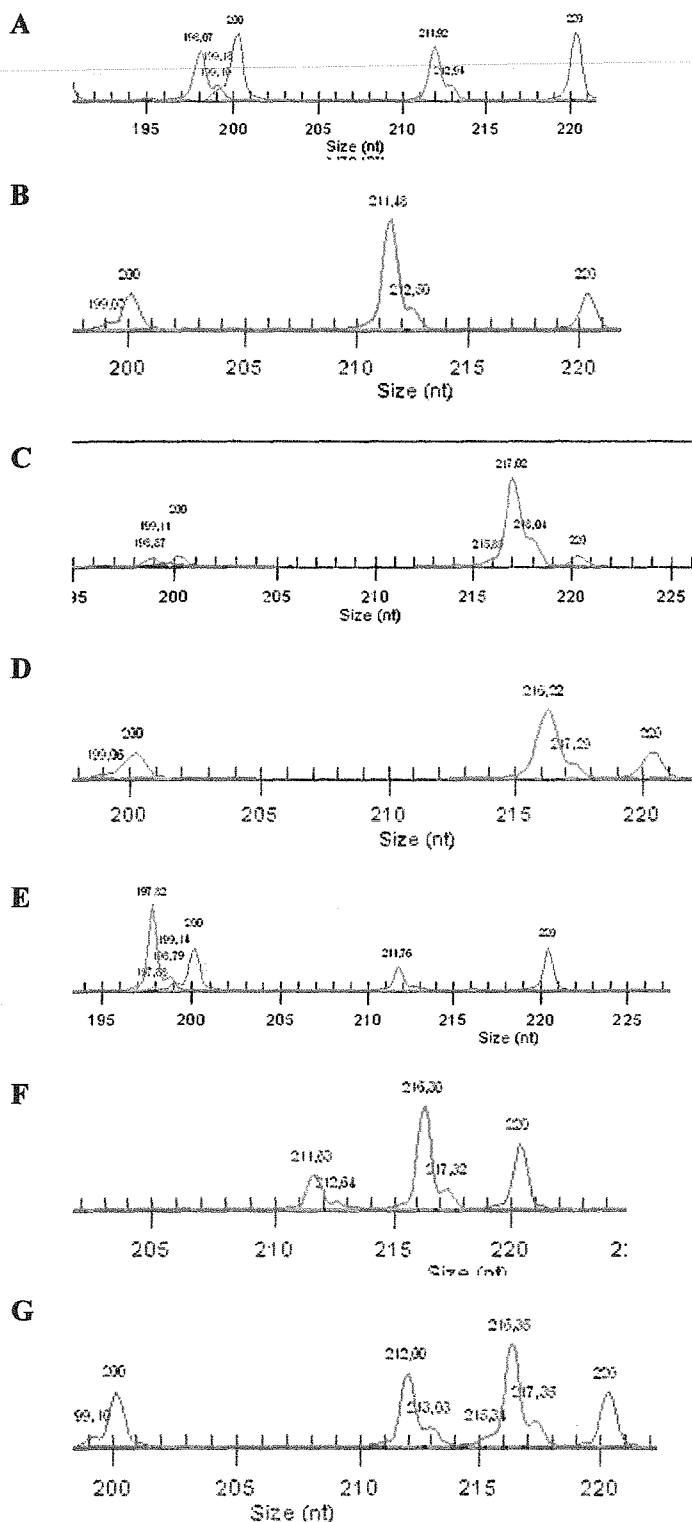
Figure 7 : Chromatogrammes obtenus suite au génotypage par électrophorèse capillaire de produits de PCR générés en utilisant le couple d'amorces microsatellites PA3 (marquage 'bleu'). Deux génotypes sont observés chez Pau (A ou B), et deux autres génotypes sont observés chez Pam , dont un « hétérozygote complexe » (C ou D). Deux génotypes « hétérozygote complexe » sont observés chez Paa (E ou F). En génotypant le produit de PCR obtenu avec PA6-F/R sur un mélange expérimental de quantités équivalentes d'ADN de Pam et de Pau , un génotype de type « hétérozygote complexe » de Paa similaire au cas F peut être créé artificiellement (G).
