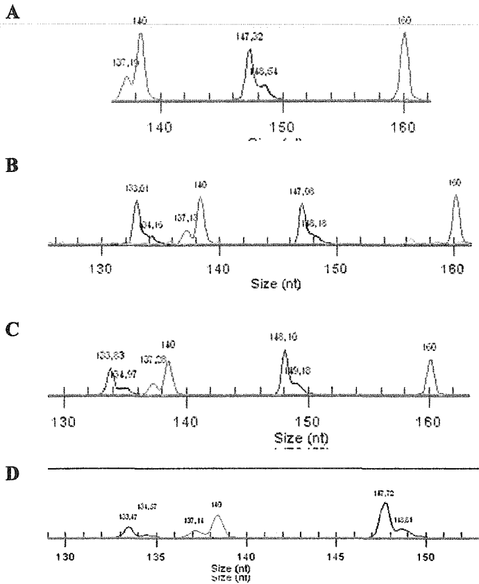
Figure 6 : Chromatogrammes obtenus suite au génotypage par électrophorèse capillaire de produits de PCR générés en utilisant le couple d'amorces microsatellites PA23 (marquage 'noir'). Un seul génotype est observé chez Pau (A), et un seul autre génotype est observé chez Pam (B). Un génotype « hétérozygote complexe » est observé chez Paa (C). En génotypant le produit de PCR obtenu avec PA23-F/R sur un mélange expérimental de quantités équivalentes d'ADN de Pam et de Pau , un génotype de type « hétérozygote complexe » ou de Paa similaire au cas C peut être créé artificiellement. (D).
