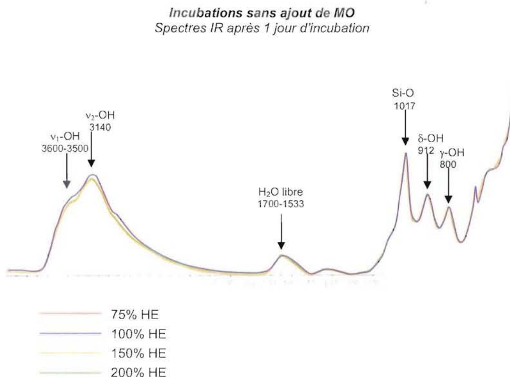
Figure 8.9 Spectres IRTF des échantillons de sol après 1 jour d'incubation sans ajout de MO.
