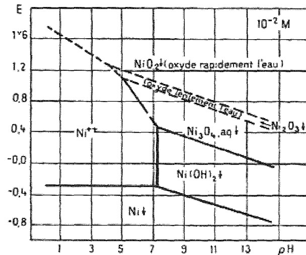
Figure 2.6 Diagramme de Pourbaix du nickel (Charlot 1983).
