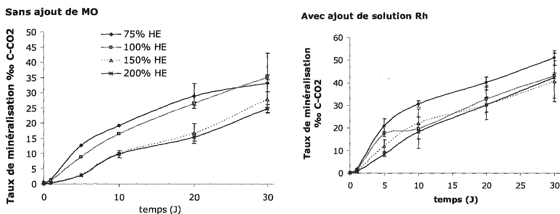
Figure 8.3 Minéralisation cumulée des matières organiques en présence de la MO autochtone du sol (à gauche) ou suite à des apports d'exsudats "rhizosphériques" modèles (à droite), exprimée en ‰ du carbone organique total initial (Indices de minéralisation, \text{C-CO}_2/\text{CO}_{10d} ).
