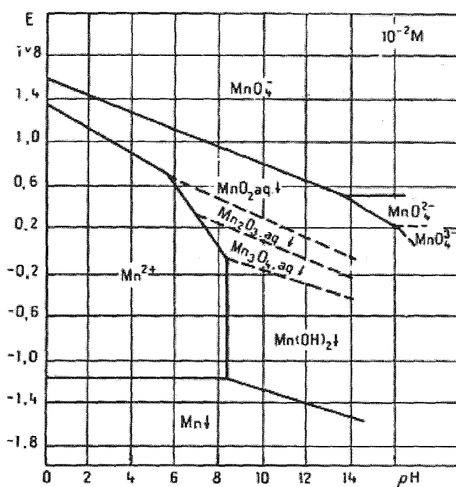
Figure 2.5 Diagramme de Pourbaix du manganèse (Charlot 1983).
