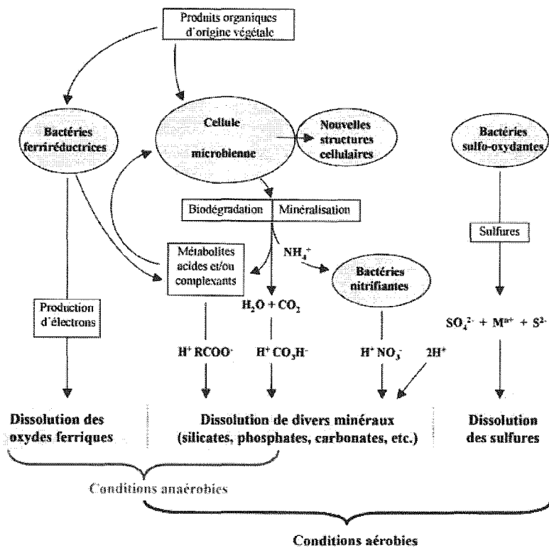
Figure 2.10 Principales interventions des microorganismes du sol sur la dissolution et l'altération des minéraux (D'après Berthelin 1998).
