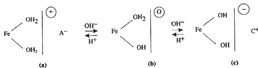
Figure 2.4 Schéma réactionnel des oxydes de fer, états et propriétés d'échange. Les traits verticaux représentent la surface d'un oxyde de fer avec des charges positives (+) en milieu acide (a), neutres (0) au point isoélectrique (b) et négatives (-) en milieu alcalin (c) (Girard et al. 2005, d'après Herbillon 1994)
