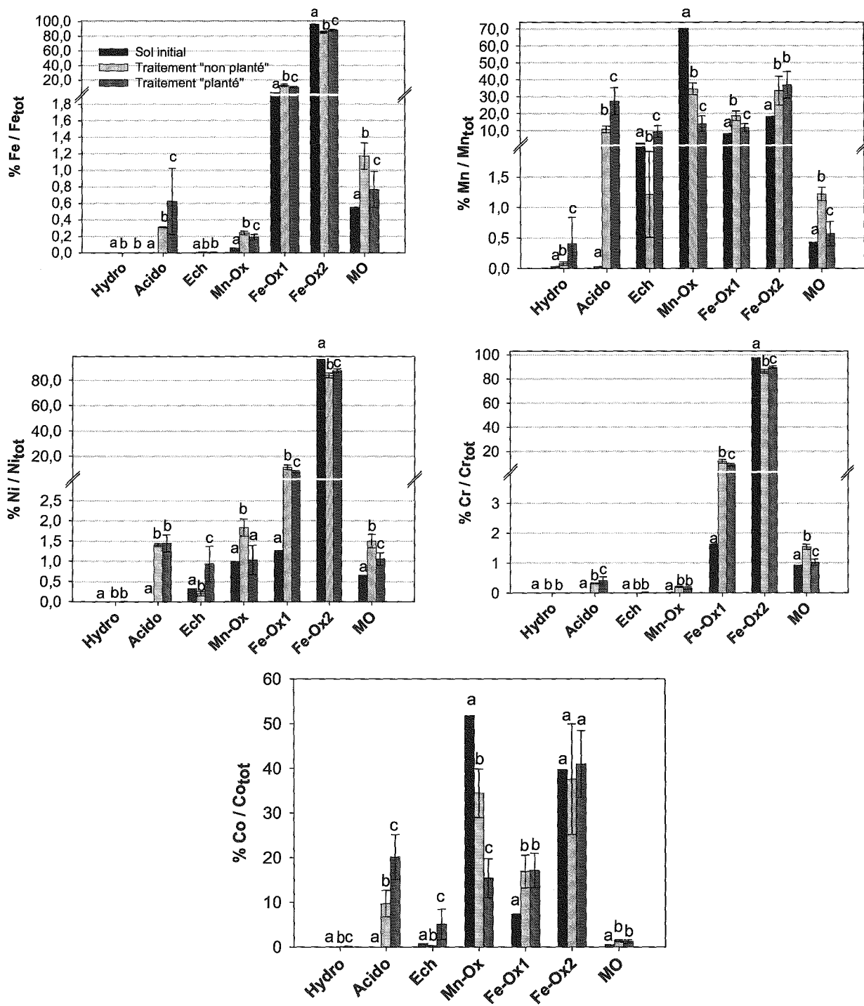
Figure 7.8 Répartition de Fe, Mn, Ni, Cr et Co dans les différents compartiments organo-minéraux et minéraux des échantillons de sol plantés ou non de maïs dans les colonnes subissant 1×8 jours d'engorgement ; les résultats présentés avec des lettres différentes (a et b) sont significativement différents (test t de Student, risque de 5%). Ces lettres sont à considérer élément par élément, et compartiment par compartiment.
