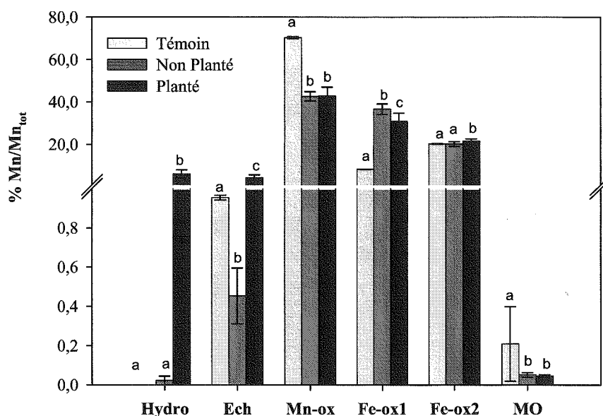
Figure 4.5 Répartition du manganèse dans les différents compartiments minéraux et organo-minéraux du support de culture 10% sol / 90% sable avant (témoin) et après incubation du substrat planté ou non de maïs.
