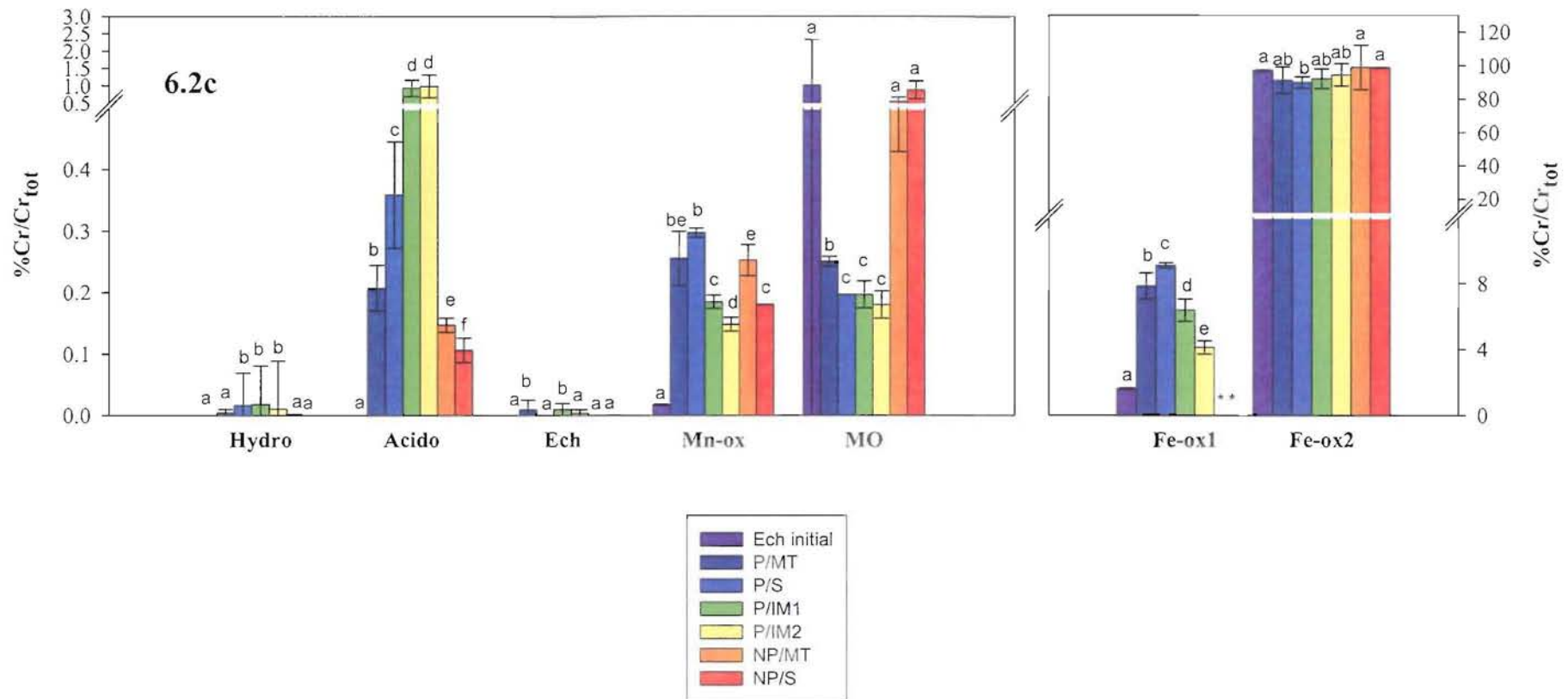
Figure 6.2c. Répartition de Cr dans les différents compartiments minéraux et organo-minéraux des échantillons de sol avant (témoin) et après incubation du substrat planté ou non de maïs (* non déterminé) ; les résultats représentés avec des lettres différentes sont significativement différents (test t de Student, risque de 5%). Les lettres sont à considérer éléments par éléments, et séparément pour chaque compartiment minéral et organo-minéral.
