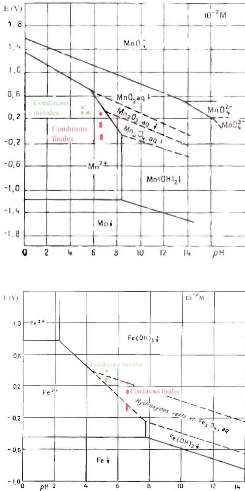
Figure 8.2 Evolution des conditions de Eh et pH des solutions de sol entre le début et la fin des incubations, vue sur le diagramme de Pourbaix du manganèse (en haut) et du fer (en bas)
