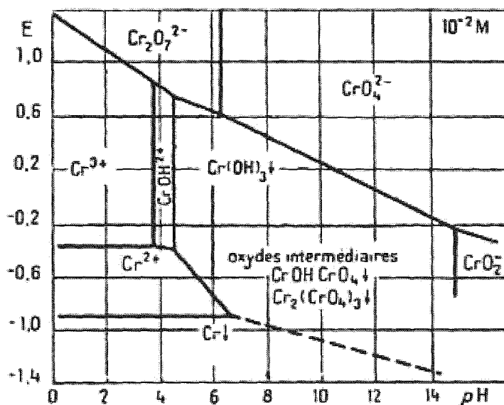
Figure 2.7 Diagramme de Pourbaix du chrome (Charlot 1983)
