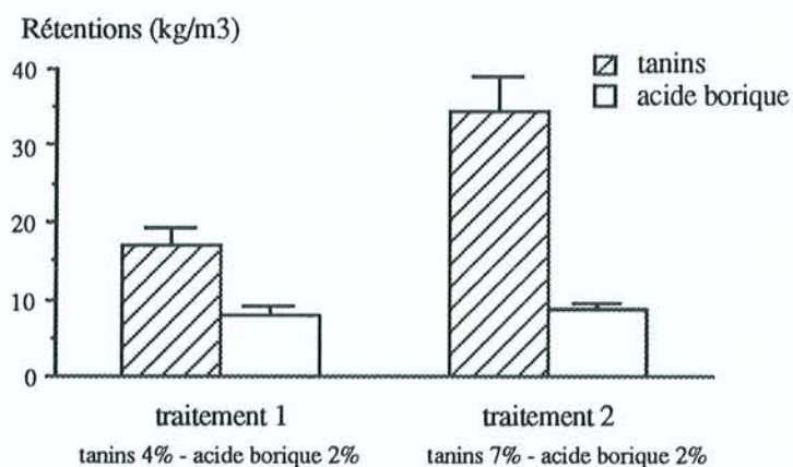
Figure 23a. Rétentions des produits de préservation dans les éprouvettes traitées par les associations acide borique-tanins (tanins : 1ère imprégnation, acide borique : 2ème imprégnation).
