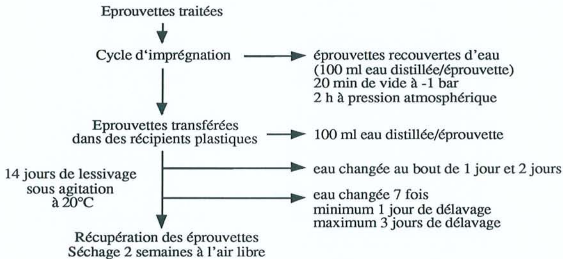
Figures 21. Etapes principales lors du délavage d'éprouvettes traitées, d'après la norme EN 84 (1979).
