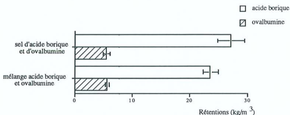
Figure 52. Rétentions d'acide borique et d'ovalbumine lors du traitement d'éprouvettes de pin sylvestre par le sel ou le simple mélange acide borique-ovalbumine.
