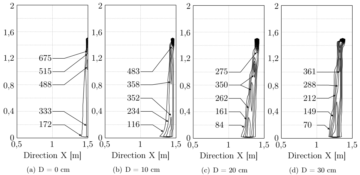
FIG. 8.15 – Évolution des fractions volumiques ( \times 10^{-6} [ \text{m}^3 d'eau / \text{m}^3 d'air]) en fonction de la configuration de la double rampe. Représentations faites selon un plan XZ passant par la buse d'injection
