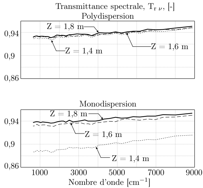
FIG. 7.24 – Évolution et comparaison des transmittances pour une monodispersion
