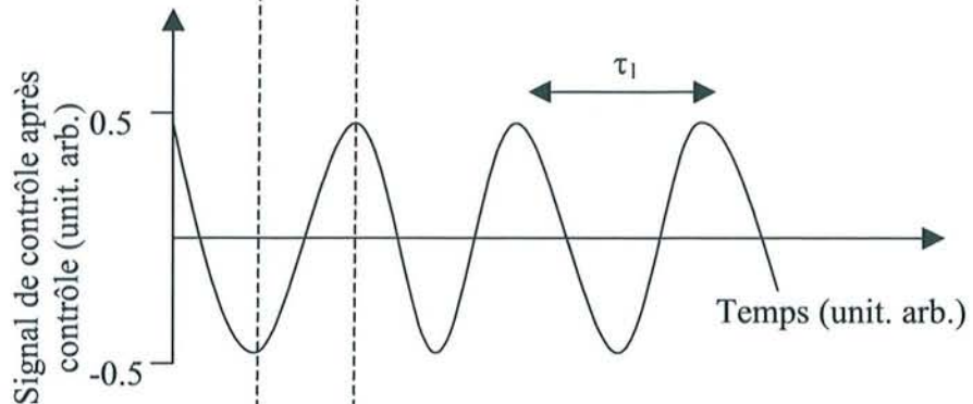
Fig. 5.14c : Signal de contrôle obtenu : (= fig. (5.14a) - fig. (5.14b)).
