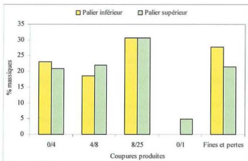
Fig. 3.25 : Bilan matière des matériaux dolomitiques de Schloss Thorn concassés et lavés sur le site de Folschette
