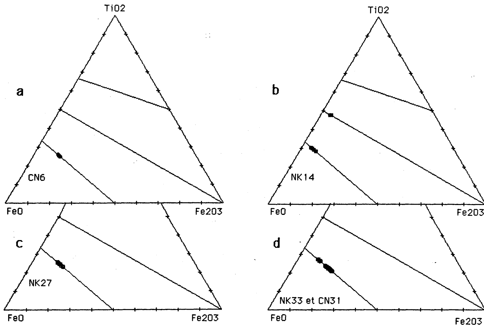
Fig. 15-25 : Compositions des oxydes des laves de la première séquence volcanique a : basalte ; b : hawaïite ; c : benmoréite ; d : trachytes hyperalcalins
