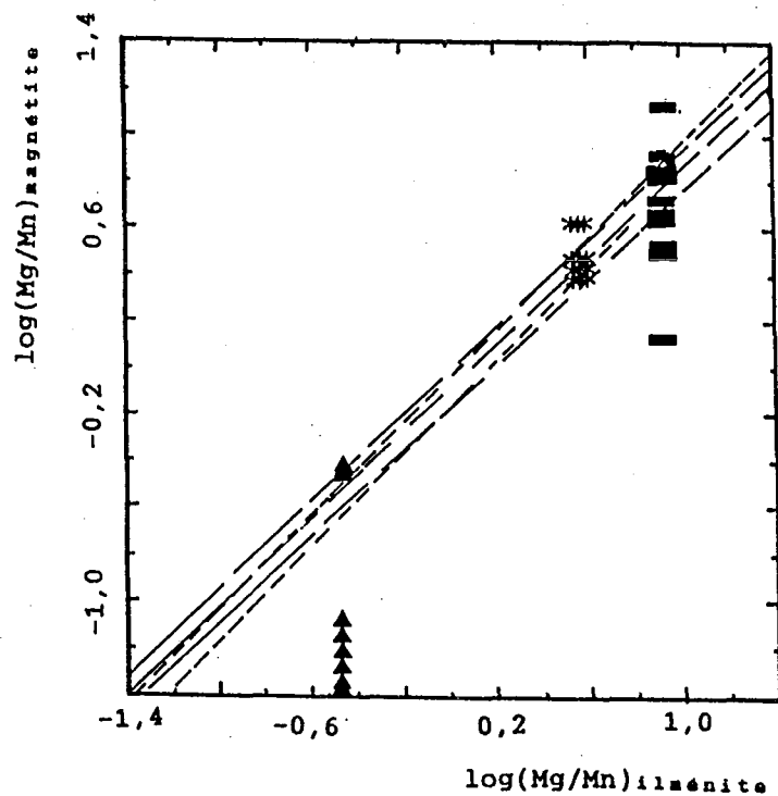
Fig. 16-12 : \log(\text{Mg}/\text{Mn})_{\text{magnetite}} en fonction de \log(\text{Mg}/\text{Mn})_{\text{ilménite}} ; test d'équilibre entre deux oxydes coexistant. Carré : hawaiites (NK4) ; astérisques : mugéarites (CN36) ; triangle : basalt de la 1ère séquence volcanique (CN4).
