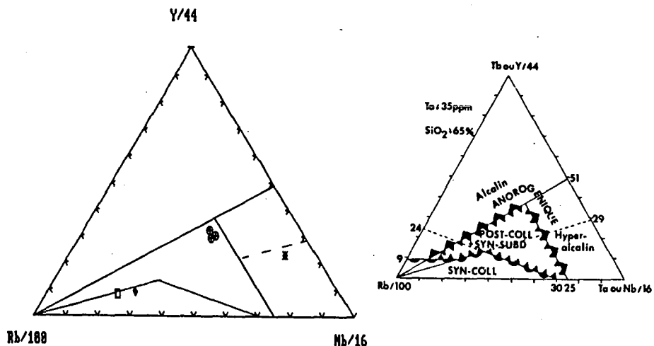
Fig. 8-3 : Distribution des granites du substratum panafricain des Monts Roupui dans le diagramme de corrélation entre les teneurs en certains éléments en traces et le site géotectonique. La grille est celle proposée par Thiéblemont et Cabanis (1990). Les granites hyperalcalins ultimes (étoile) sont aussi reportés. Carré vide et losange plein : granite à biotite et muscovite secondaire ; cercle avec croix : granite à amphibole et biotite.
