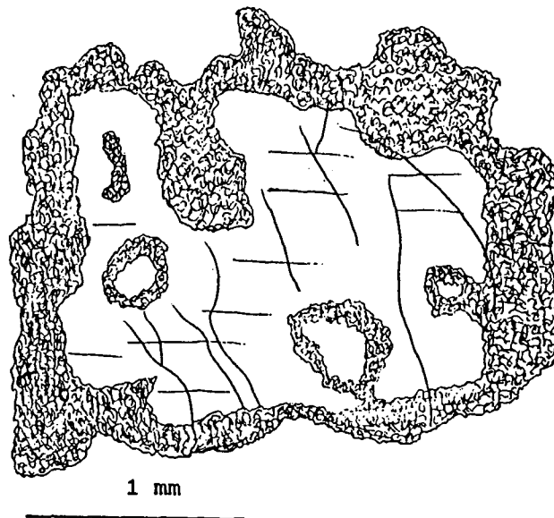
Fig. 12-4 : Xénocrystal de feldspath alcalin montrant une frange de fusion trempée à l'éruption.
