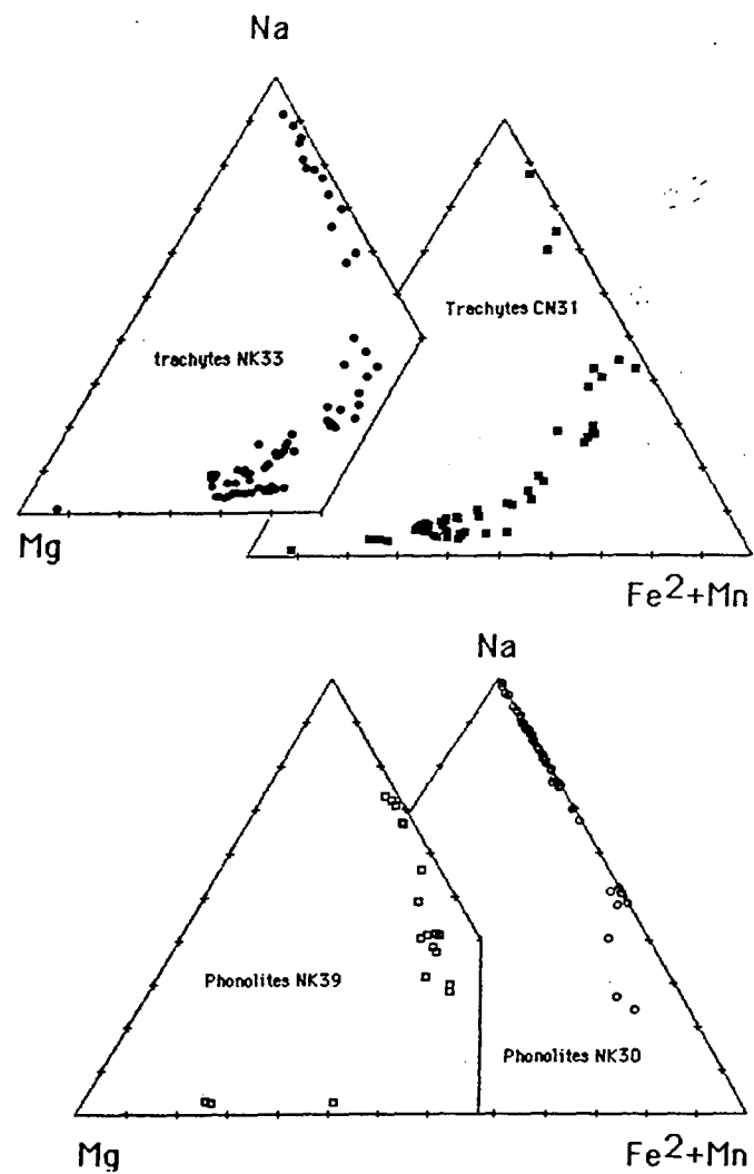
Fig. 15-11 : Evolution des compositions des pyroxènes sodiques
