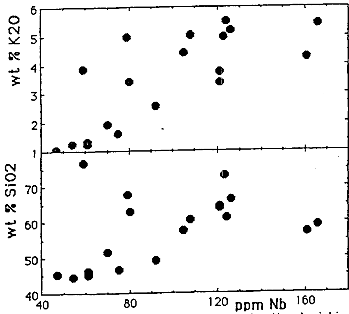
Fig. 18-3: Variations des éléments majeurs en fonction du niobium.
