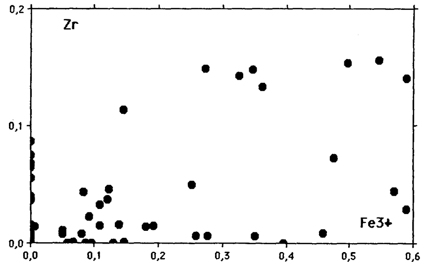
Fig. 15-17' : Zr en fonction de Ti (haut) ou Fe 3+ (bas) :
