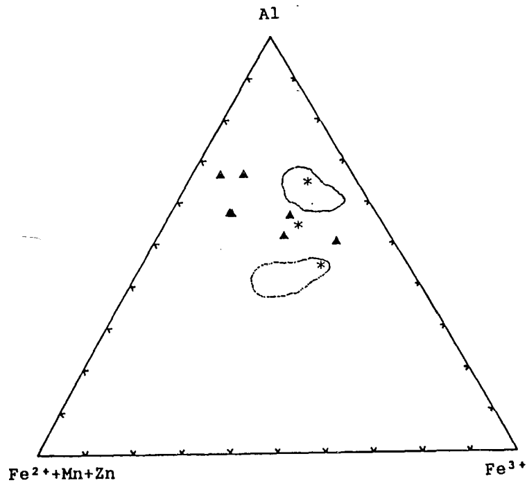
Fig. 6-6 : Diagramme \text{Al} - (\text{Fe}^{2+} + \text{Mn} + \text{Zn}) - \text{Fe}^{3+} (moles %) des Sr-ménilites du Mont Etinde ; triangle : cette étude ; astérisque : Fitton et Hughes (1981). Les domaines des Sr-ménilites des néphélines du Maroc central (Velde et Rachdi, 1988) sont représentés.
