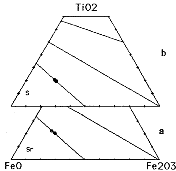
Fig. 6-4b : Oxydes des néphélinites à méllite (a) et des hæÿnophyres (b)
