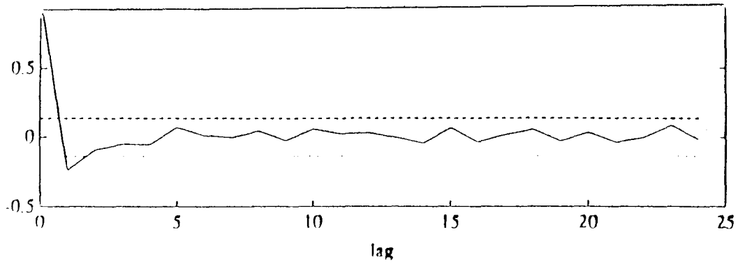
Figure 8.1 : Fonction d'autocorrélation des résidus du modèle de Tco
