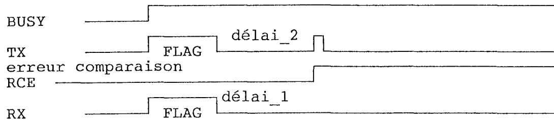
figure 19 : émission avec un écart de moins de 125 nanosecondes et avec des délais DELAI_DAD identiques.
