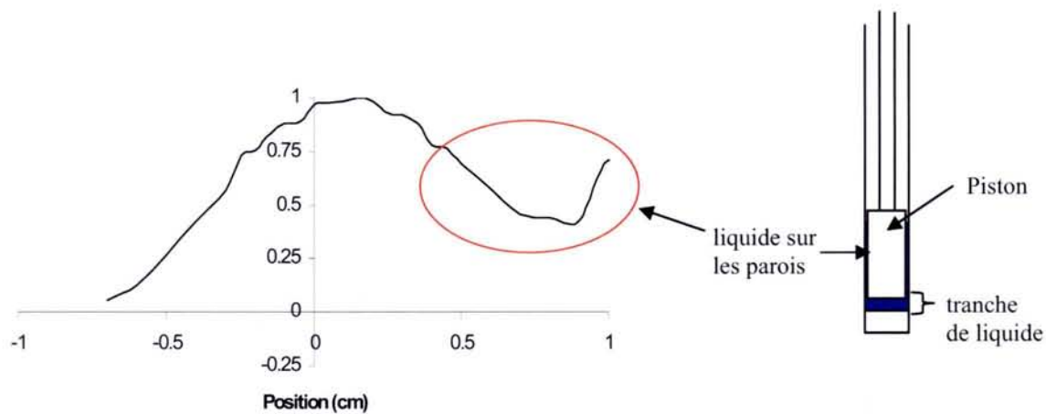
Figure 2.13 : Profil expérimental (à gauche) du champ radiofréquence émis par une bobine en selle de cheval de 8 mm de hauteur, pour une tranche de 1mm d'eau. La partie droite du profil est faussée par le liquide situé entre le piston et les parois du tube (schéma de droite)
