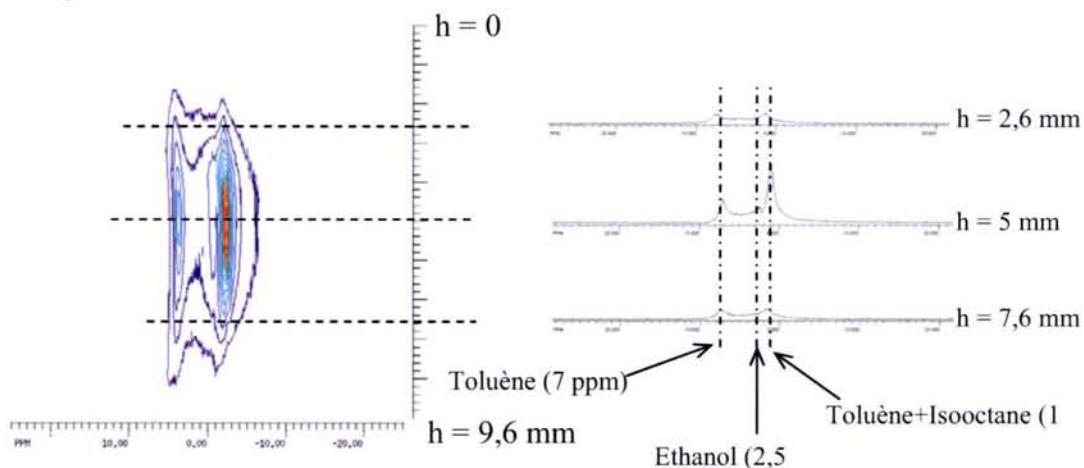
Figure 2.36 : Carte de déplacement chimique obtenue avec un échantillon prélevé dans la zone de soudure d'un flacon de PeHD en contact avec le carburant modèle pendant 6 semaines à 40°C. A droite, les spectres correspondant aux zones les plus représentatives
