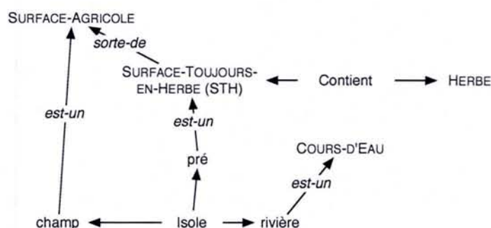
FIG. 1.1 – Un exemple de réseau sémantique représentant la phrase « Le pré isole le champ de la rivière ». Les concepts génériques sont étiquetés en majuscule, les concepts individuels en minuscule. Les relations entre concepts sont en italique.
