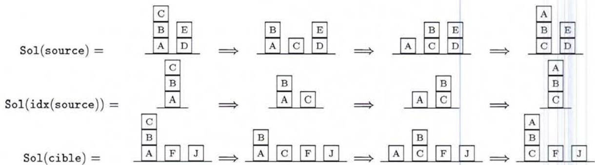
FIG. 2.4 – Un exemple d’adaptation à l’aide d’un chemin de similarité reposant sur une classification dure. La double flèche \Rightarrow indique les transitions entre les différents états du processus de résolution. On sait comment inverser A et C dans source, on adapte pour le faire dans cible.
