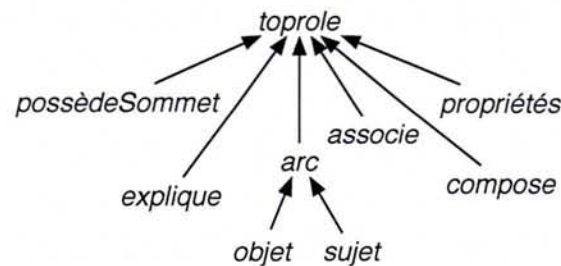
FIG. 5.2 – Hiérarchie des rôles \mathcal{H}_R utilisés pour la représentation des connaissances dans notre système.
