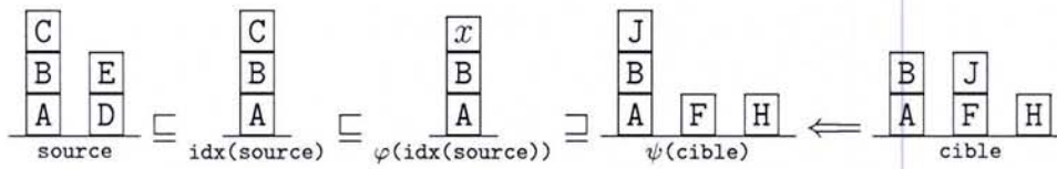
FIG. 2.5 – Un exemple de chemin de similarité obtenu après classification élastique. Le bloc étiqueté par x correspond au bloc générique qui peut être substitué par tout autre bloc.
