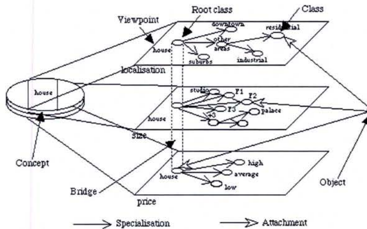
FIG. 1.4 – Le concept de MAISON (HOUSE) d'une base de connaissance TROEPS. Figure tirée de [48].
