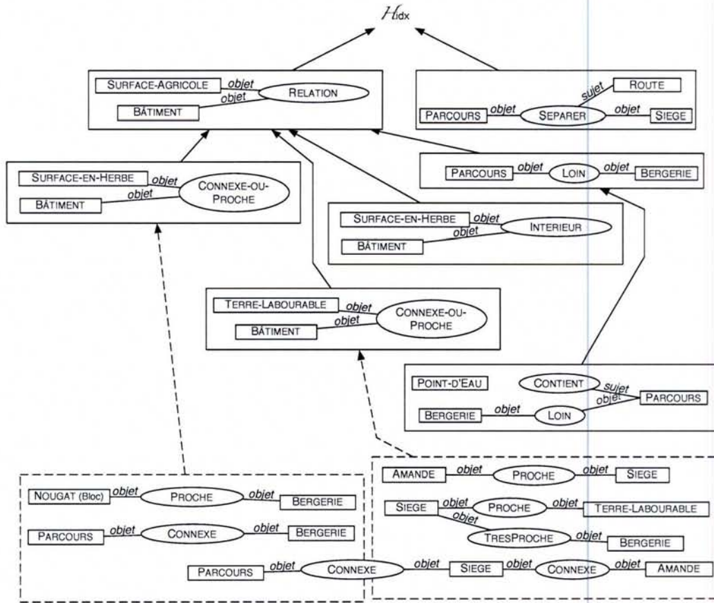
FIG. 5.4 – Hiérarchie partielle des index de cas (les explications ne sont pas représentées).
