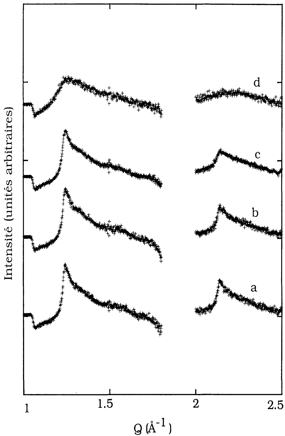
Figure IV.9: Spectres correspondant à 1,05 monocouche
