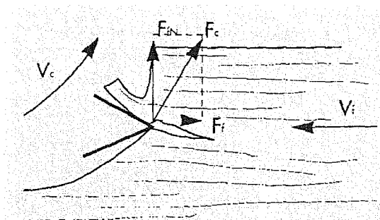
Figure II.29 3 ème phase - fendage (d'après Koch, 1964)
