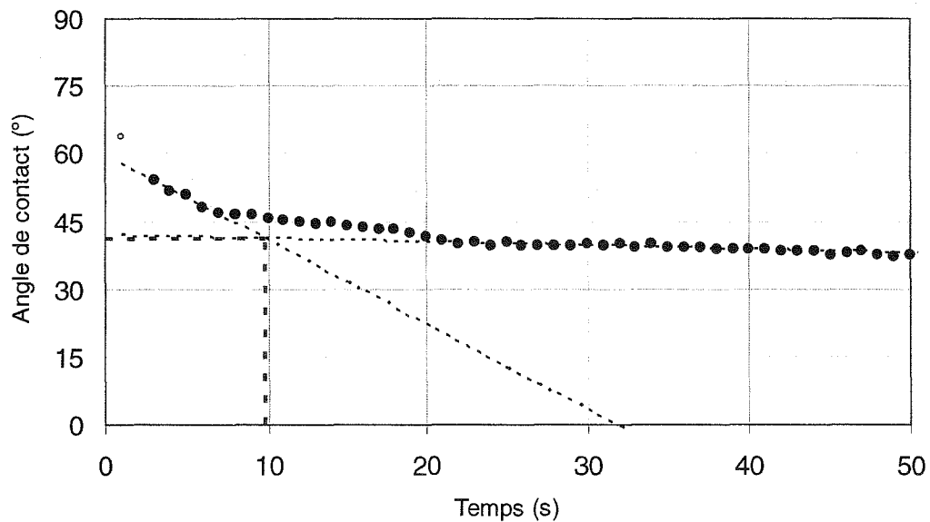
Figure III.16 Exemple de la détermination de l'angle d'équilibre pour une éprouvette de hêtre (N3-essai 9, après 12 jours)
