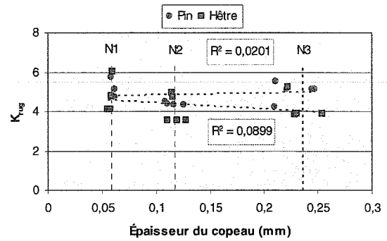
Figure IV.81 - Influence du niveau d'usinage sur le K_{rug} (critère de rugosité)
