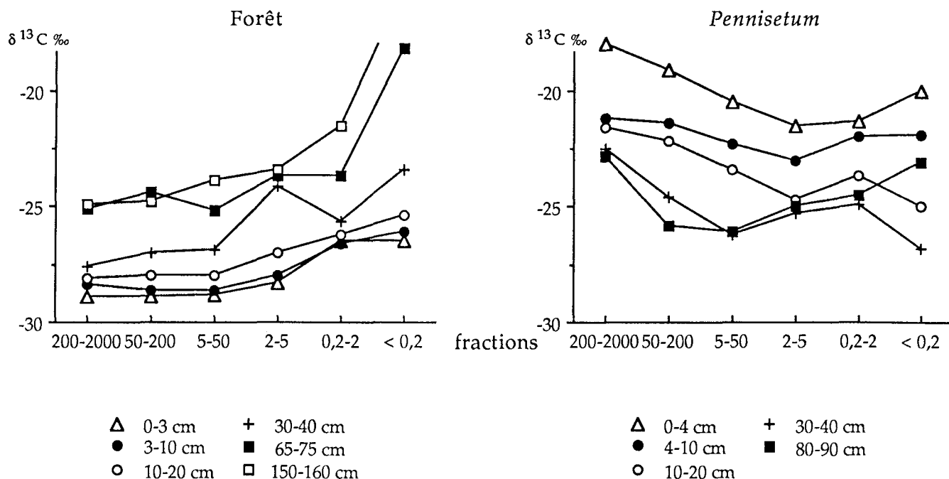
Figure 23.- Valeurs de \delta^{13}\text{C} des fractions granulométriques du sol sous forêt et du sol sous Pennisetum .
