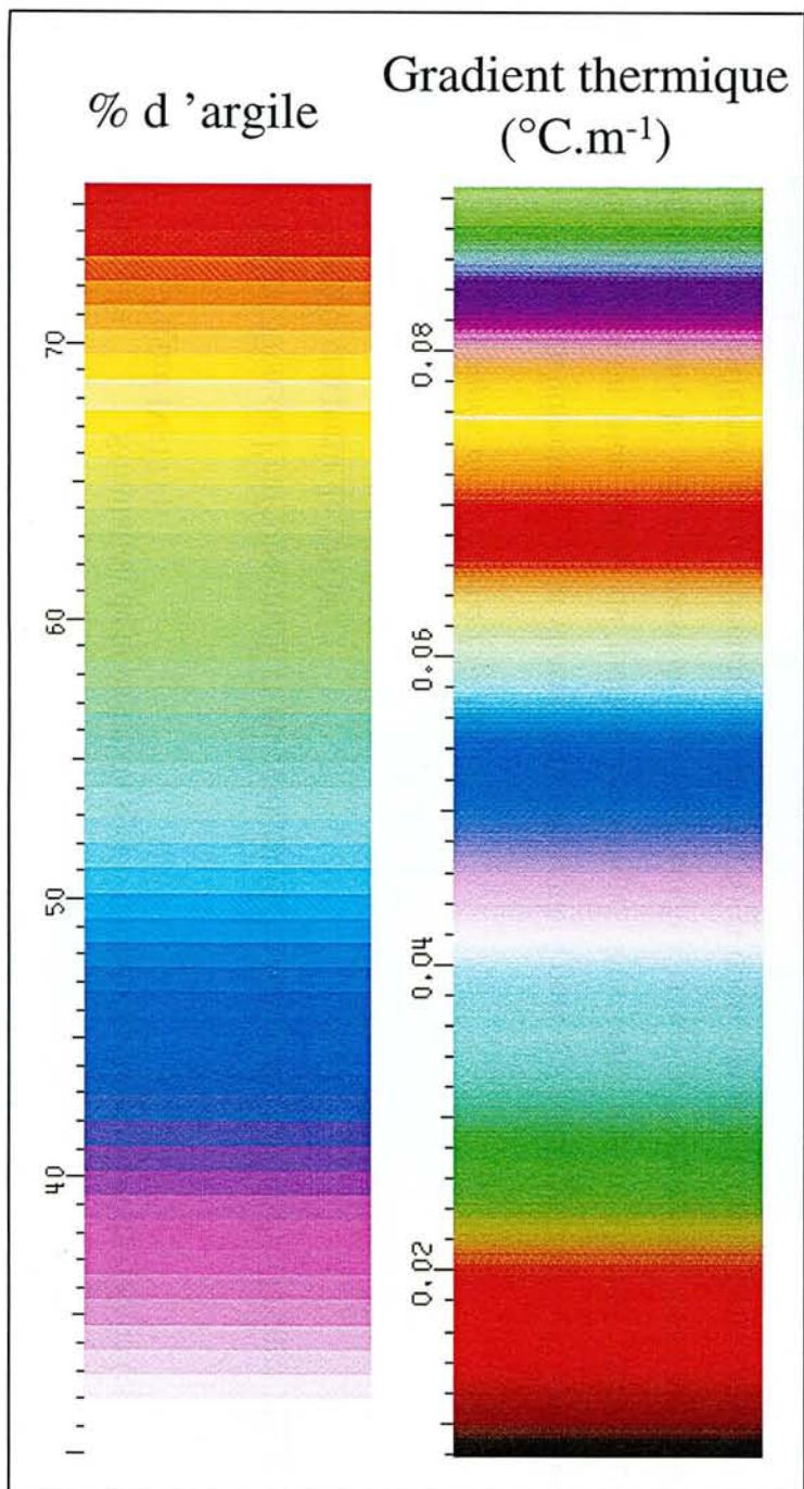
Figure IV.17: Gradients thermiques simulés pour H2 dans l'espace (x,y = t, z); (échelle * 15); A, B, C, ..., S sont les codes alphabétiques des noms des sondages. Les sphères représentent le pourcentage d'argilosité.
