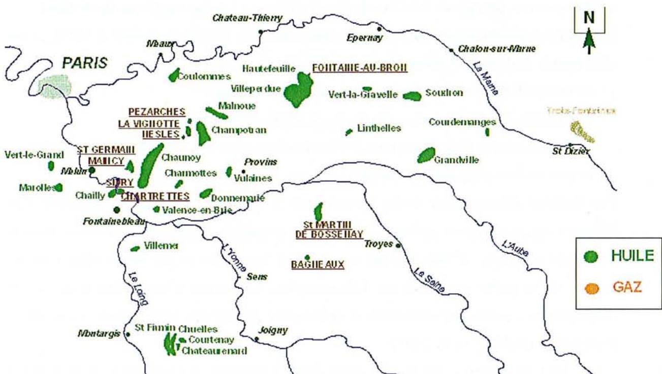
Figure II-4 : Gisements principaux du bassin de Paris
