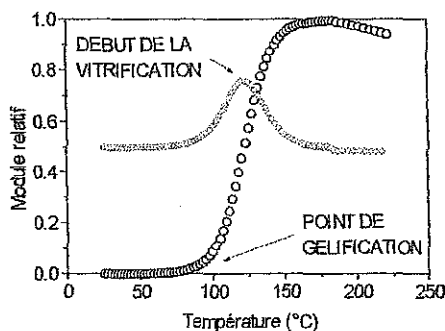
Figure 5.9 : Représentation schématique du module relatif lissé (o) de résines phénoliques et de sa dérivée (◇).
