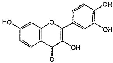
Figure 1.14 : fisétine
