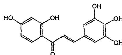
Figure 1.20 : robtéine
