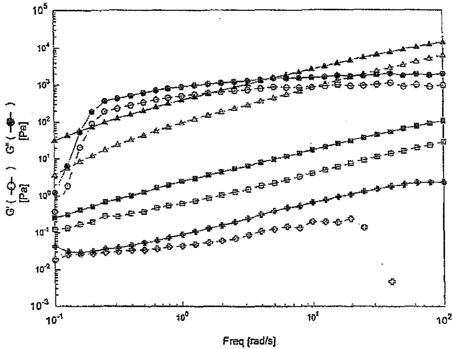
Figure 2.7 : Variations au cours du balayage en fréquence à amplitude de déformation constante \gamma = 10\% des modules élastiques et visqueux G' (○) et G'' (●) des solutions aqueuses d'extrait de tannin de pin pour des concentrations de 20% (✚), 30% (■), 40% (●) et 50% (▲)
