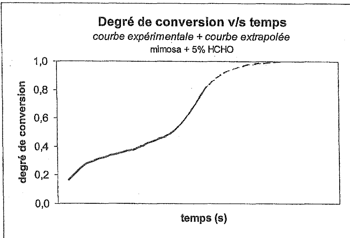
Figure 3.15 : Représentation graphique des limitations de la méthode utilisée pour le calcul du degré de conversion après le point de gel, avec en trait plein la courbe expérimentale, et en pointillés la courbe théorique.
