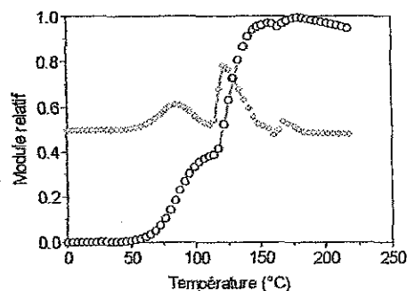
Figure 5.10 : Représentation schématique du module relatif (o) de résines phénoliques et de sa dérivée (◇).
