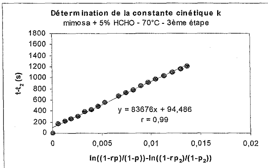
Figures 3.16 (a), (b) et (c) : Détermination graphique des constantes cinétiques k des trois réactions successives de type second ordre qui caractérisent la polycondensation avant le point de gel du tannin de mimosa avec 5% HCHO à 70°C.
