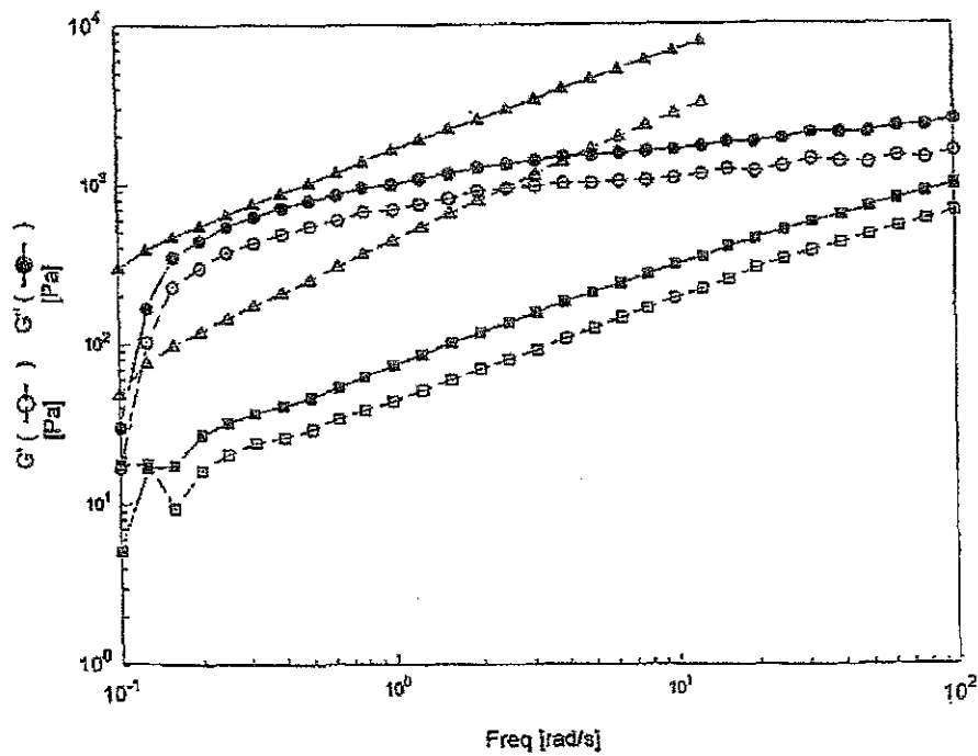
Figure 2.8 : Variations au cours du balayage en fréquence à amplitude de déformation constante \gamma = 10\% des modules élastiques et visqueux G' (○) et G'' (●) des solutions aqueuses d'extrait de tannin de pécan pour des concentrations de 30% (■), 40% (●) et 50% (▲)
