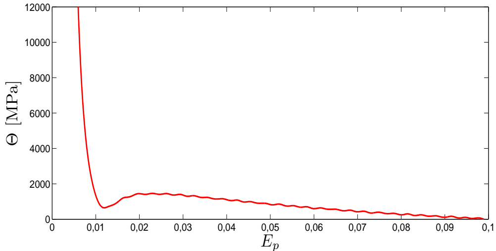
(b) Evolution du taux d'écroissage en fonction de la déformation plastique
