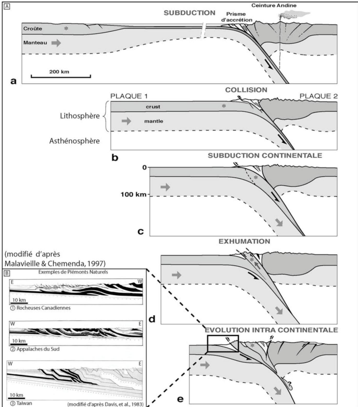
Figure III.2.1 : A : Schéma de l'évolution d'une chaîne de montagnes de collision. a ) Phase de subduction d'une croûte océanique, ce qui engendre la création d'un prisme d'accrétion et initie une ceinture orogénique
