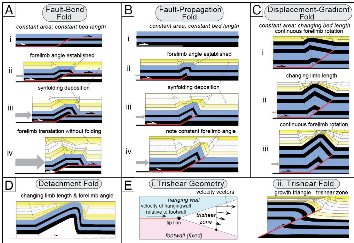
Figure II.5.1 : Synthèse des principaux types de modèle de plissement (Burbank & Anderson, 2001)
