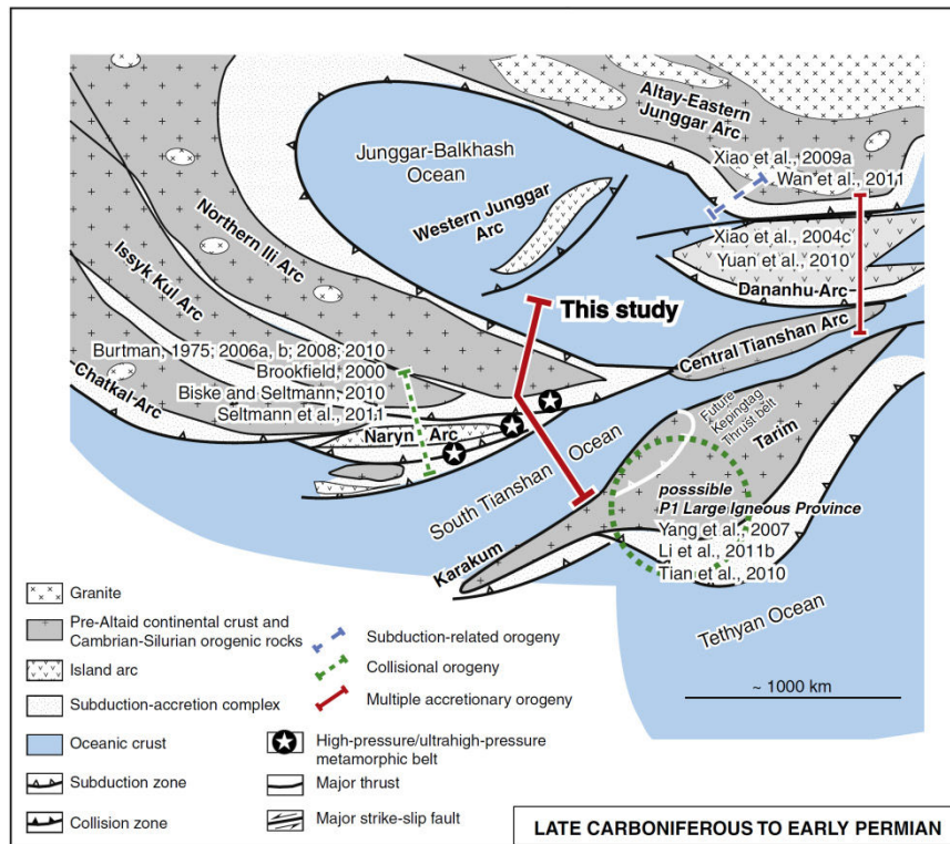
Figure III.2 : Paléogéographie du Tianshan oriental au Carbonifère supérieur / Permien inférieur (Xiao et al. , 2013).
