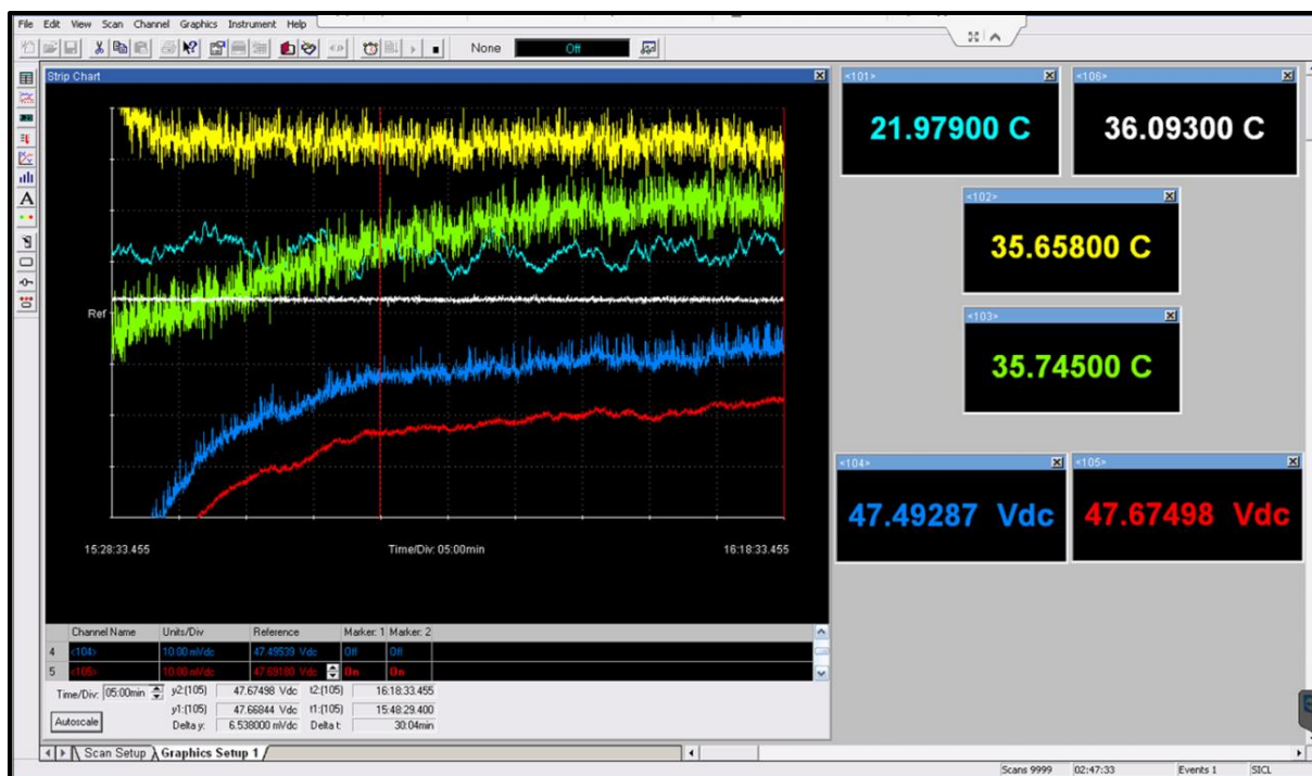
Figura 30. Proceso de estabilización de la desorción de gas metano a una temperatura promedio de 35°C.
