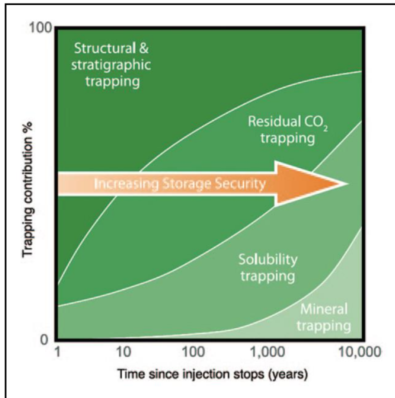
Figura 2. Mecanismos de retenção de CO 2 em função do tempo. (ICCP 2005)
