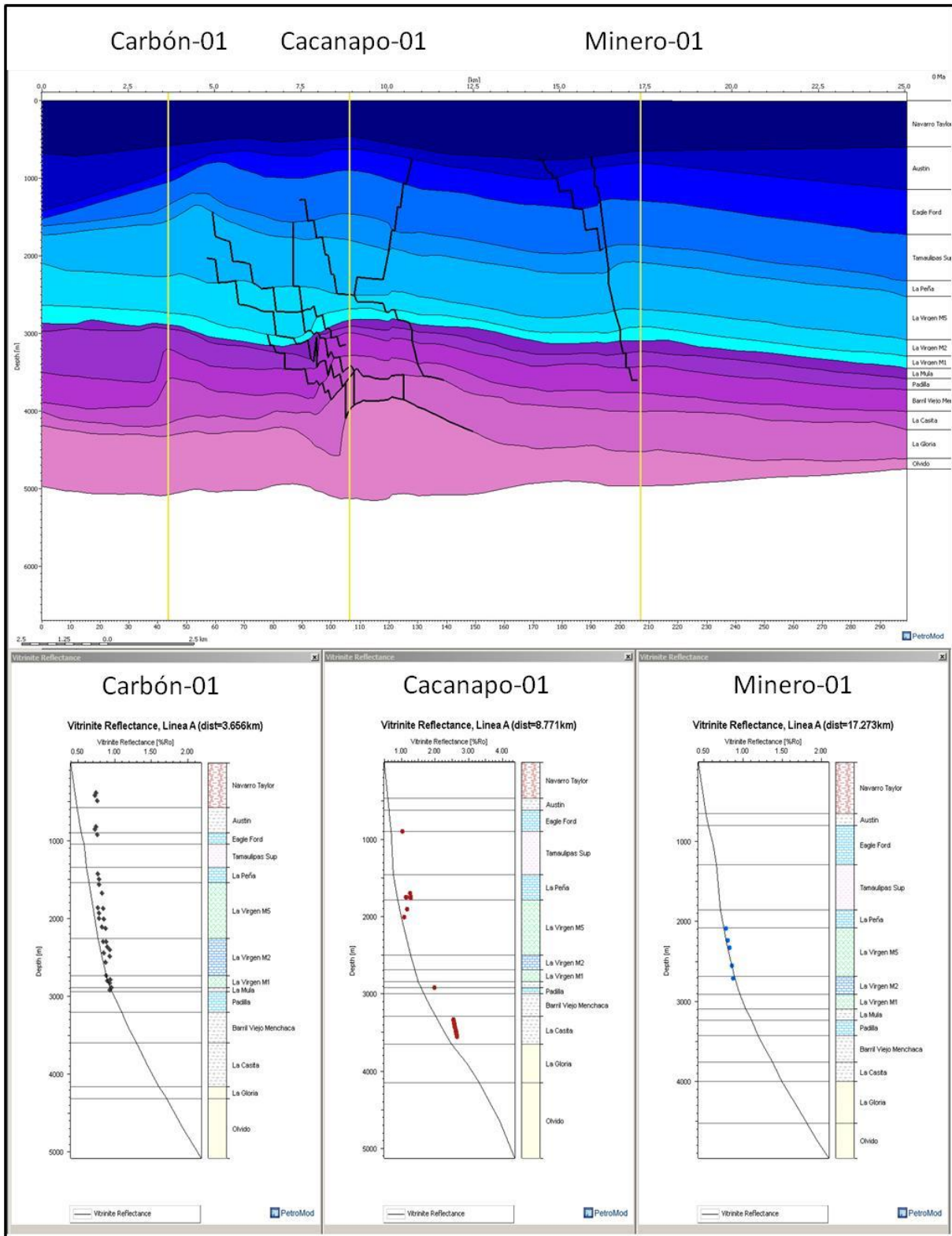
Figura 91. Extracción de pozos para la calibración termocinética con reflectancia de la vitrinita %Ro. de los pozos Cacanapo-101, Merced-01 y Ulua-01.
