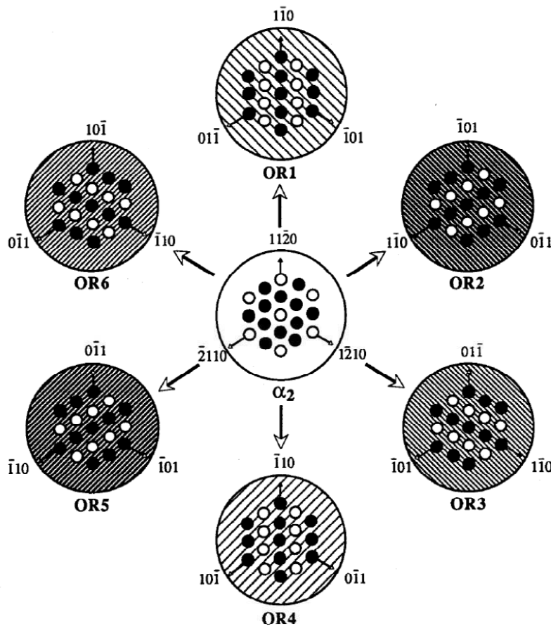
Figure I-4 : Représentation des différents variants issus de la relation d'orientation de Blackburn. Reproduction de Zghal et col. [ZGHAL 1997].
