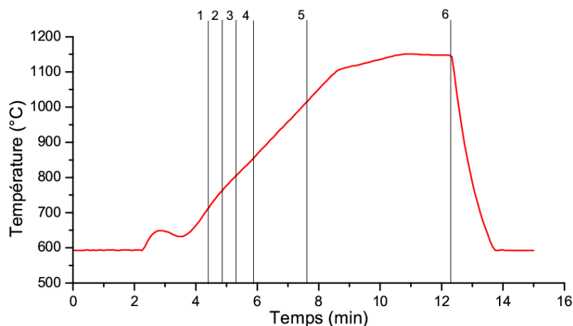
Figure IV-1 : Cycle standard de densification jusqu'à 1150°C. Températures depuis lesquelles certains cycles ont été interrompus.
