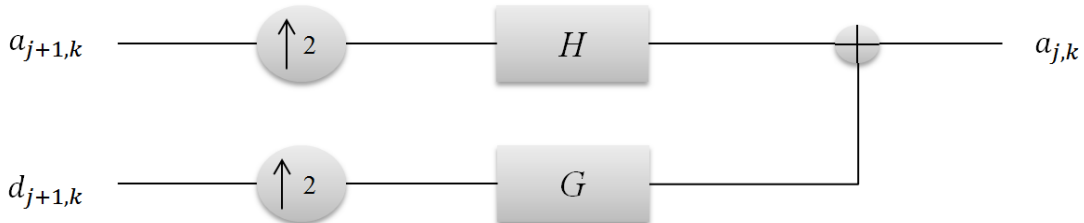
Figure 72 : Bloc de reconstruction à l'aide de filtres passe-haut et passe-bas
