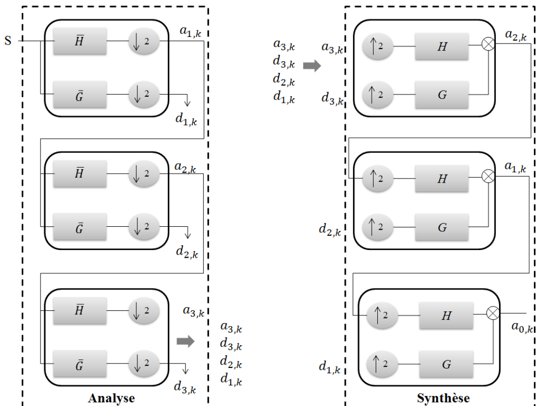
Figure 73 : Analyse et synthèse à l'échelle 3 par bancs de filtres
