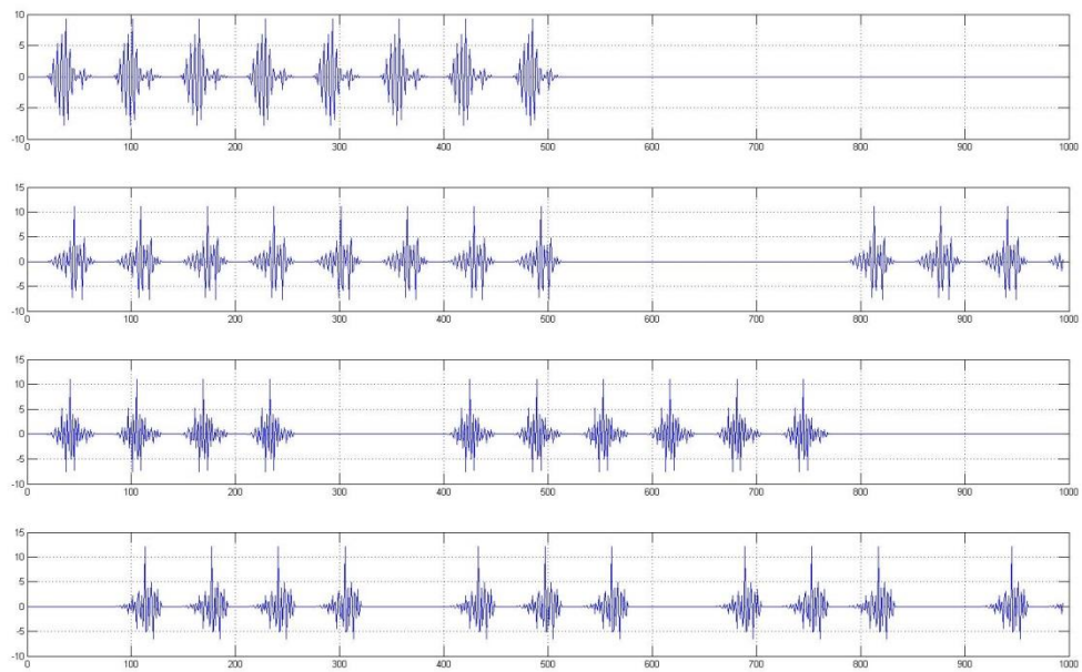
Figure 96 Exemple de trains d'impulsions au niveau 4 pour les entrées 13,14, 15 et 16, ondelette Daubechies 2
