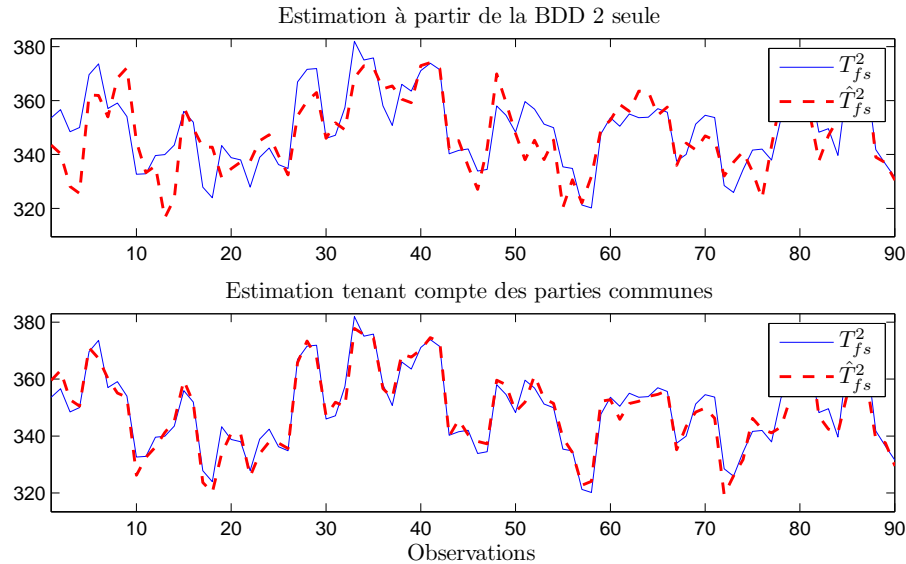
FIGURE 4.11 – Evolution de T_{fs}^2 et ses estimées, sur les données de test, avec l'ancien (table 4.7) et le nouveau (table 4.10) modèle
