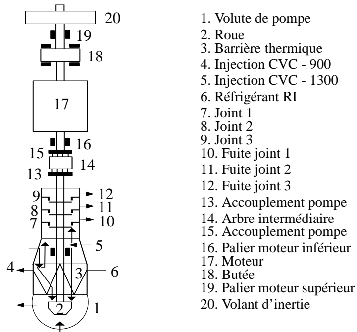
FIGURE 4.1 – Schéma d'un GMPP
