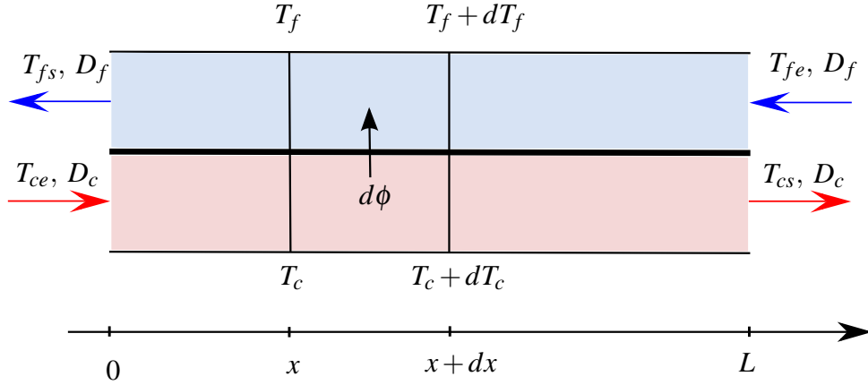
FIGURE 4.9 – Élément d'échangeur de longueur dx
