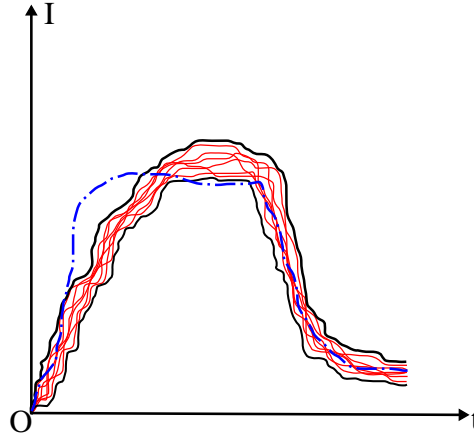
FIGURE 1.5 – Trace de normalité délimitée par les deux courbes noires et, en trait discontinu, la courbe du courant électrique d'un actionneur en défaut
