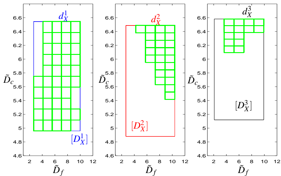
FIGURE 4.18 – Domaines de variation des variables d'entrée aboutissant aux sorties de modèles non discernables
