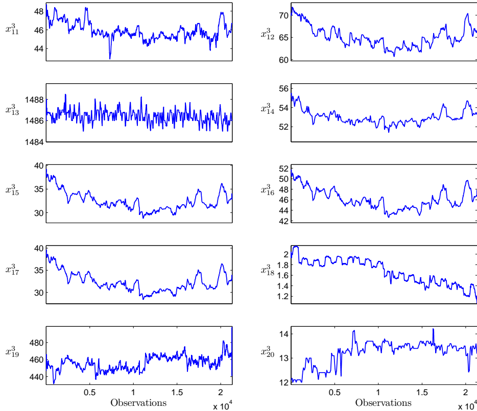
FIGURE 4.4 – Evolution des variables mesurées sur la pompe 1
