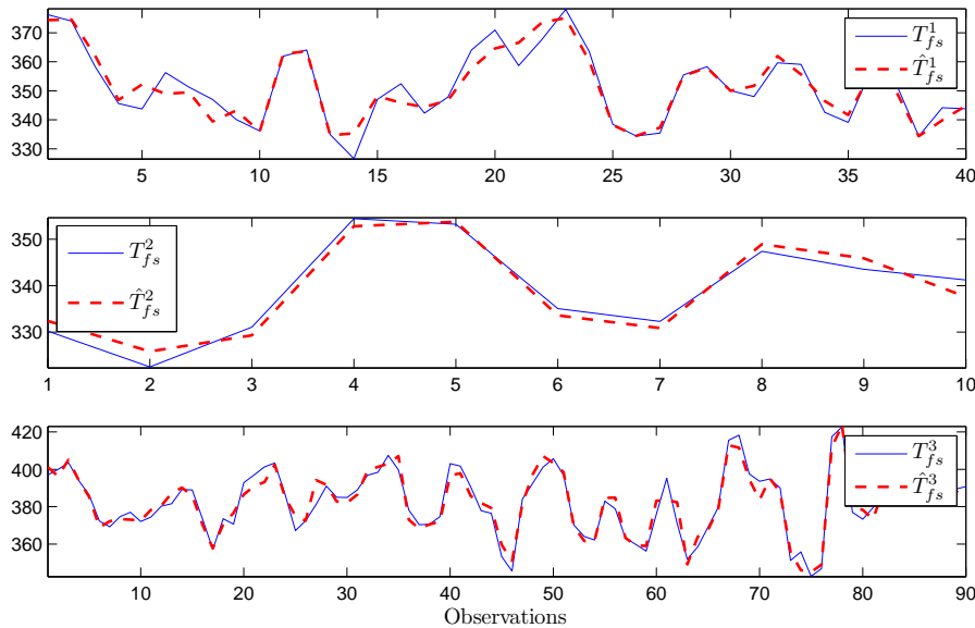
FIGURE 4.10 – Evolution des variables T_{fs}^q , q = 1, 2, 3 et leurs estimées par les modèles identifiés sur chaque base de données indépendamment les unes des autres
