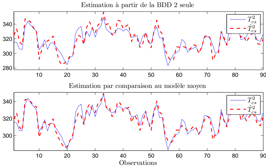
FIGURE 4.14 – Evolution de T_{cs}^2 et son estimée, sur les données de test, par le modèle identifié à partir de la BDD2 seule et celui sous contraintes de proximité à un modèle moyen
