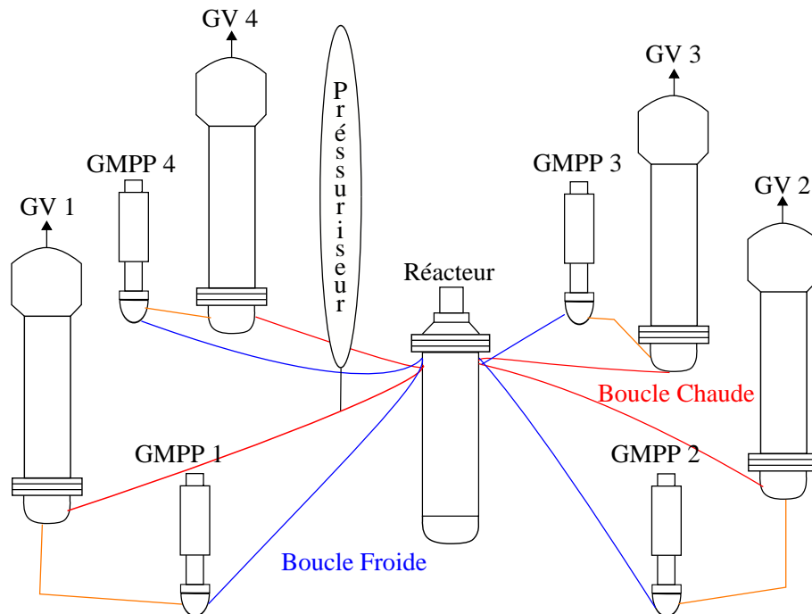
FIGURE 4.2 – Système étudié
