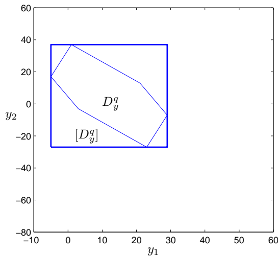
FIGURE 3.4 – Pavé [D_Y^q] circonscrit au domaine D_Y^q
