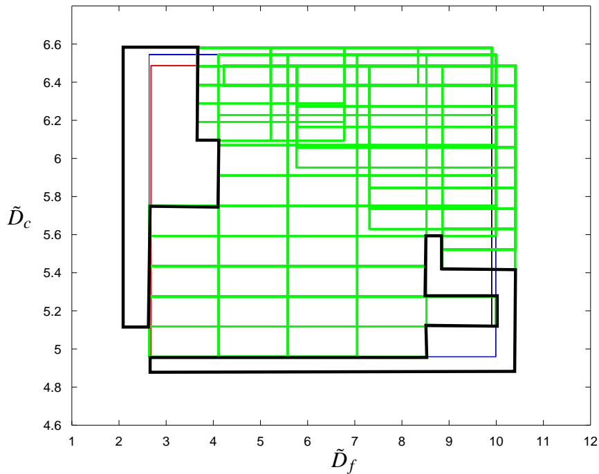
FIGURE 4.19 – Domaine (délimité par le trait noir épais) des variables d’entrée garantissant la discernabilité des sorties des modèles
