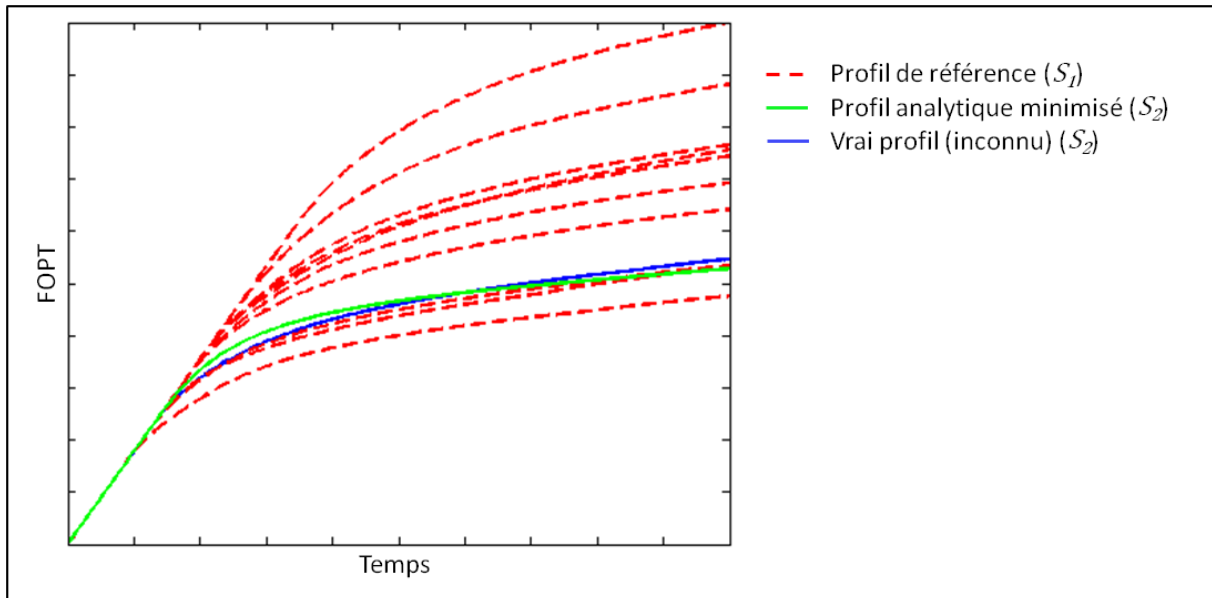
Figure 28 : Exemple de profil minimisé. Les courbes rouges, représentent les courbes de référence de \mathcal{S}_1 qui ont servi pour la minimisation, la courbe verte correspond au profil analytique résultat de la minimisation, et la courbe bleue au profil obtenu grâce au simulateur d'écoulements pour le même modèle.
