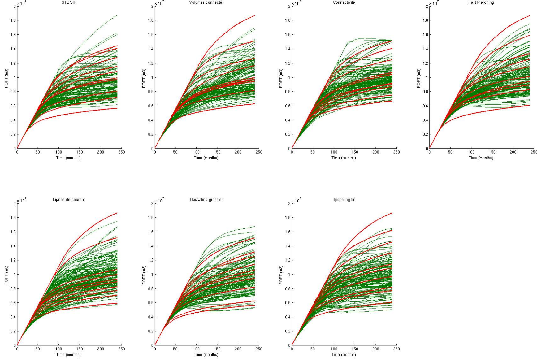
Figure 53 : Ensemble de profils obtenus pour chaque proxy. Les courbes rouges représentent ceux obtenus par simulation dynamique et les courbes vertes, ceux obtenus par minimisation.
