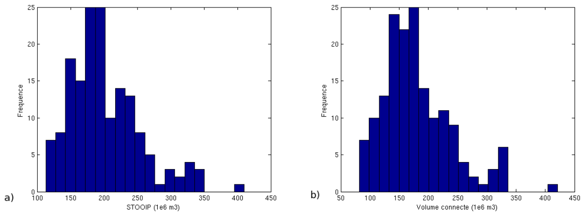
Figure 42 : Histogramme des résultats des proxys (a) STOPIP et (b) Volume connecté.
