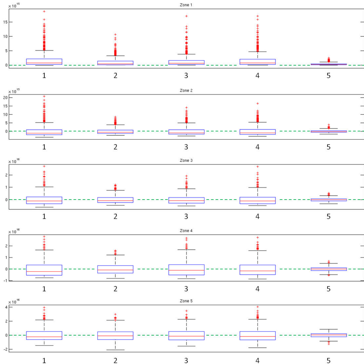
Figure 61 : Distributions des résidus par zone pour les proxys (1) STOIP, (2) Volumes connectés, (3) Connectivité, (4) Fast Marching et (5) Upscaling.
