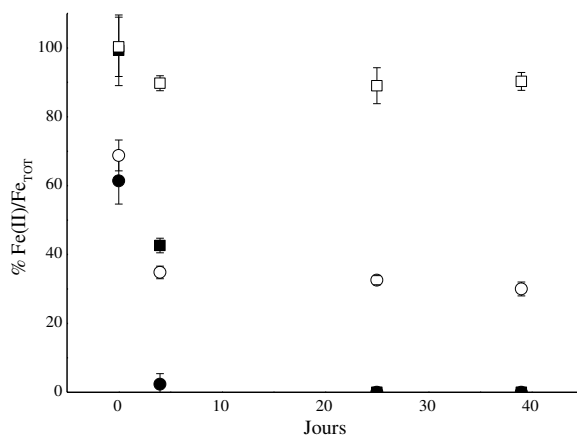
Figure 13: Évolution du ratio Fe(II)/Fe TOT au cours des incubations Fe(II) soluble - souche TIE-1 (carré noir), Fe(II) soluble seul (carré blanc), de la rouille verte carbonatée - souche TIE-1 (rond noir) et de la rouille verte carbonatée seule (rond blanc).
