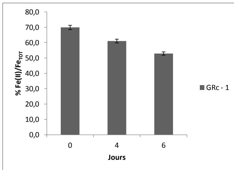
Figure 10: Évolution du ratio \text{Fe(II)/Fe}_{\text{TOT}} de la rouille verte carbonatée incubé en présence de BoFeN1.
