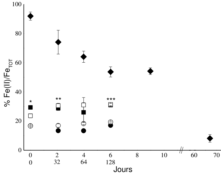
Figure 9: Évolution du ratio \text{Fe(II)/Fe}_{\text{TOT}} avec BoFeN1 en présence de : Fe(II) soluble (◆), minerai de fer intact (■), sidérite naturelle (●). Les symboles vides correspondent aux contrôles abiotiques (sans bactéries) en présence de minerai de fer intact (□) et de sidérite naturelle (○). Sur l'abscisse, le premier axe (en haut) correspond au temps de réaction de BoFeN1 avec le Fe(II) soluble et le second (bas) avec le minerai de fer intact et la sidérite. Pour les incubations avec les minerais (valeurs valables pour minerai de fer intact et sidérite), les concentrations en nitrates et nitrites ont été suivies par dosage colorimétrique instantané (bandelettes QUANTOFIX®): *, [\text{NO}_3^-] \approx 30 \text{ mM} et [\text{NO}_2^-] \approx 0 \text{ mM} ; **, [\text{NO}_3^-] \approx 15 \text{ mM} et [\text{NO}_2^-] \approx 0 \text{ mM} et ***, [\text{NO}_3^-] \approx 0 \text{ mM} et [\text{NO}_2^-] \approx 0 \text{ mM} . Dans les témoins, les concentrations en nitrates et nitrites sont constantes au cours du temps avec [\text{NO}_3^-] \approx 30 \text{ mM} et [\text{NO}_2^-] \approx 0 \text{ mM} .
