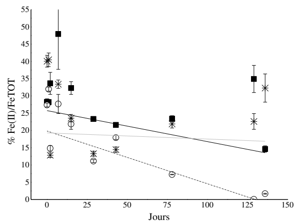
Figure 6: Évolution du ratio Fe(II)/Fe TOT au cours du temps de la suspension de sidérite dans le milieu AtF (pH 3). Condition microaérobie = carrés noirs et pente - trait continu noir; Condition aérobie = ronds blancs et pente - trait pointillé noir; Condition aérobie sans agitation = étoiles et pente - trait continu gris. Le tableau rend compte du % Fe(II) oxydé par jour (pente) seulement si le résultat de l'ANOVA (analyse de la variance, p-value) est inférieur à 0,05. Si p-value > 0,05 alors la pente n'est pas significativement différente de 0 (pas d'oxydation).
